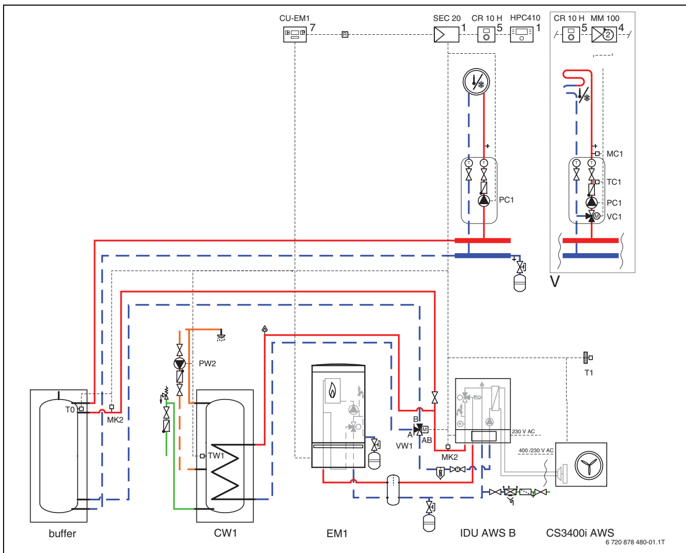
Afb. 39 Buiteneenheid met binneneenheid en twee cv-circuits
