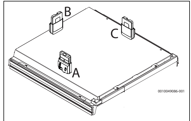
Afb. 29 Bevestigen van de houder op de bovenmantel van de binneneenheid. Naast de houder, toont de afbeelding ook de Draadloze module welke zich in de houder bevindt
