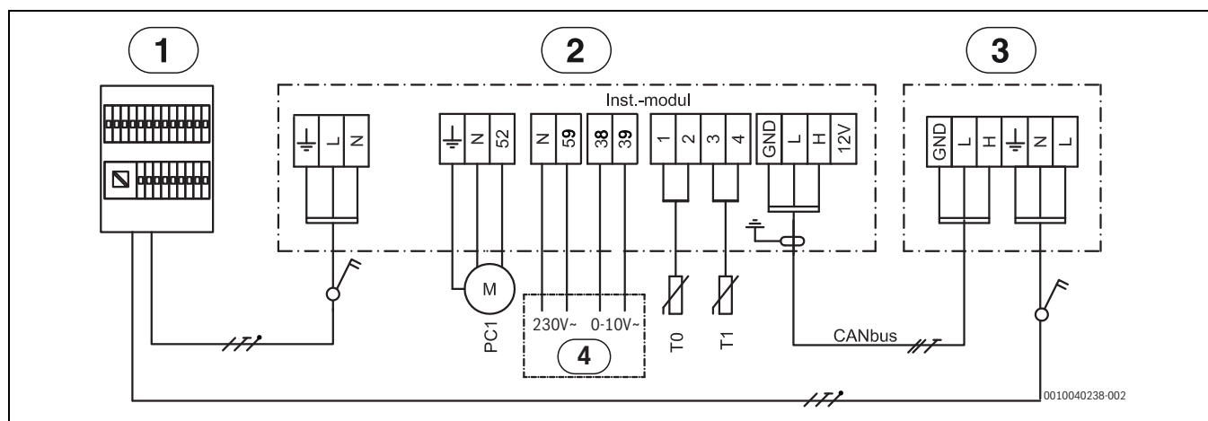
Afb. 42 Elektrisch schema
