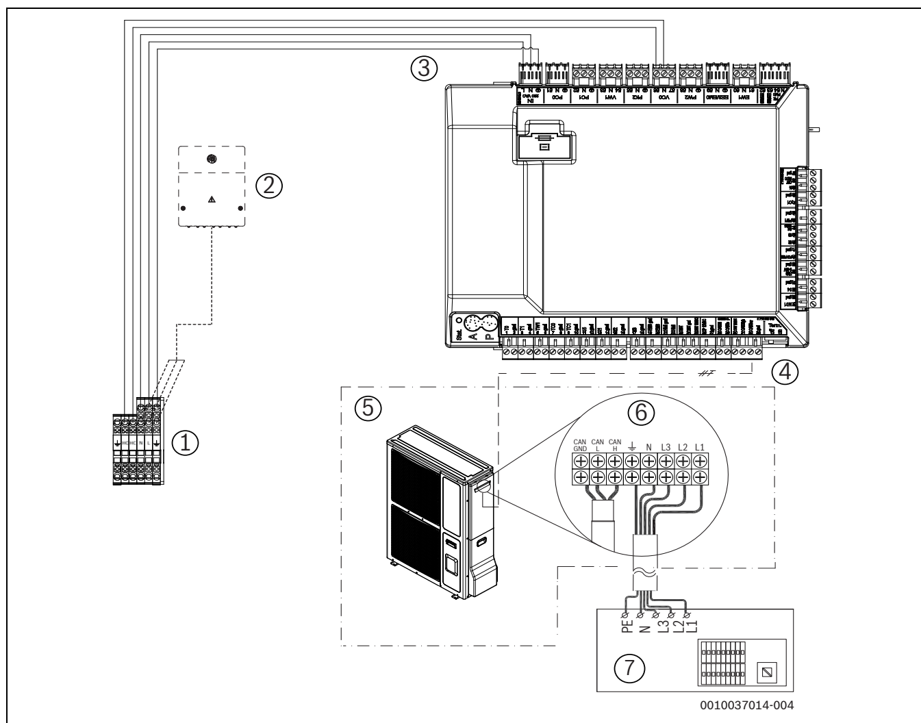
Afb. 45 Binneneenheid met 400 V 3N ~ buiteneenheid
