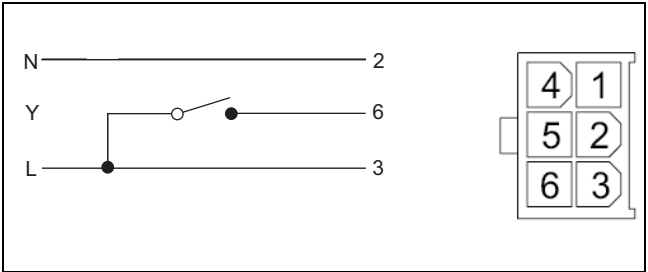
Afb. 23 Molex-stekker
