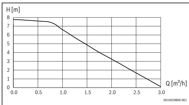
Afb. 32 Capaciteitscurve van de primaire circulatiepomp (PCO)
