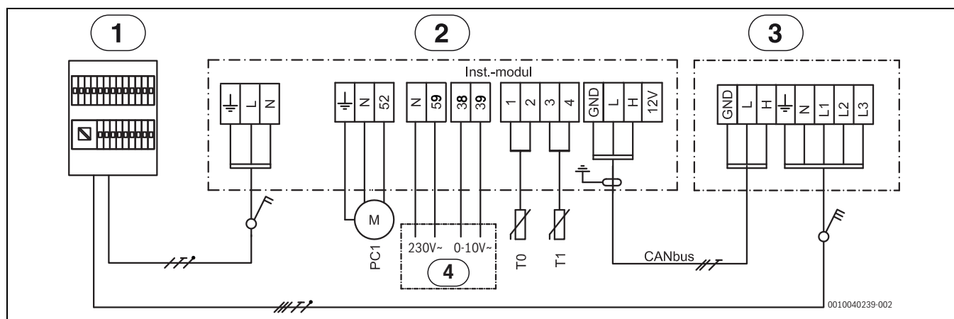
Afb. 43 Elektrisch schema
