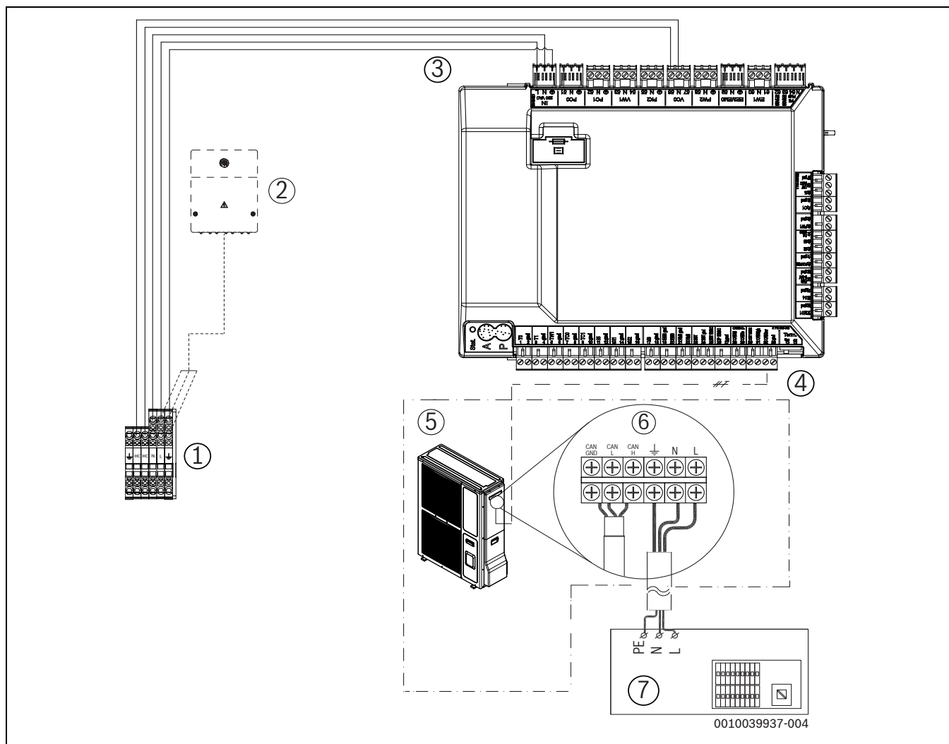
Afb. 44 Binneneenheid met 230 V~ buiteneenheid
