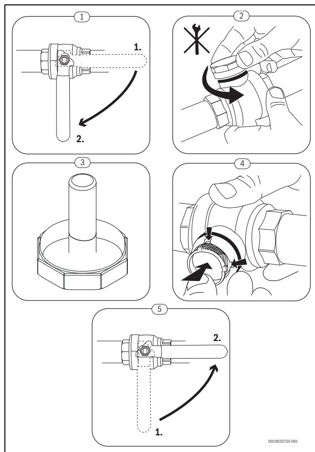
Afb. 19 Deeltjesfilter reinigen
