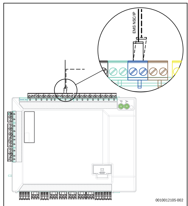
Fig. 20 Raccordement EMS sur le module d'installation
