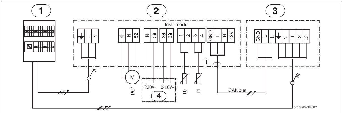
Fig. 43 Schéma de câblage
