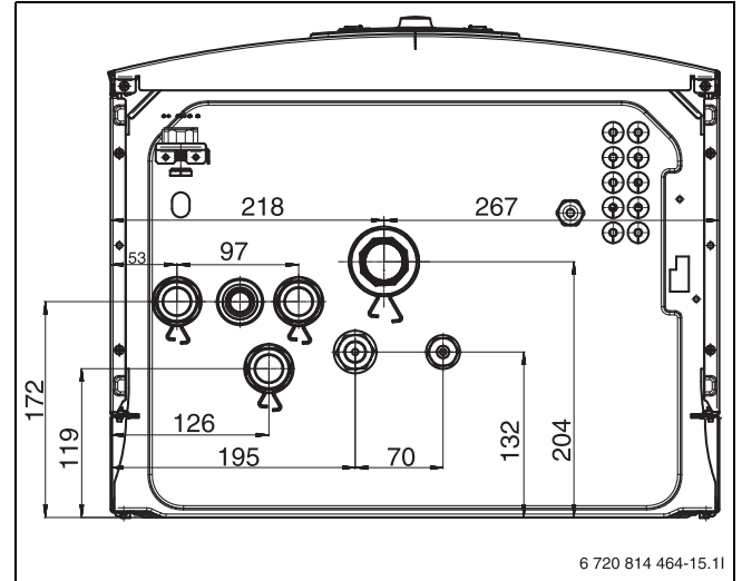
Fig. 5 Dimensions et raccordements
