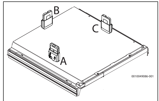
Fig. 29 Fixer le support sur la partie supérieure de l'appareil sur pieds. En plus du support, la figure indique également Module radio qui se trouve à l'intérieur du support
