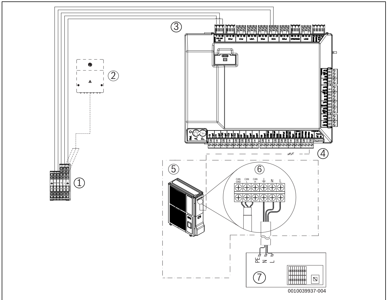
Fig. 44 Unité intérieure avec unité extérieure 230 V~
