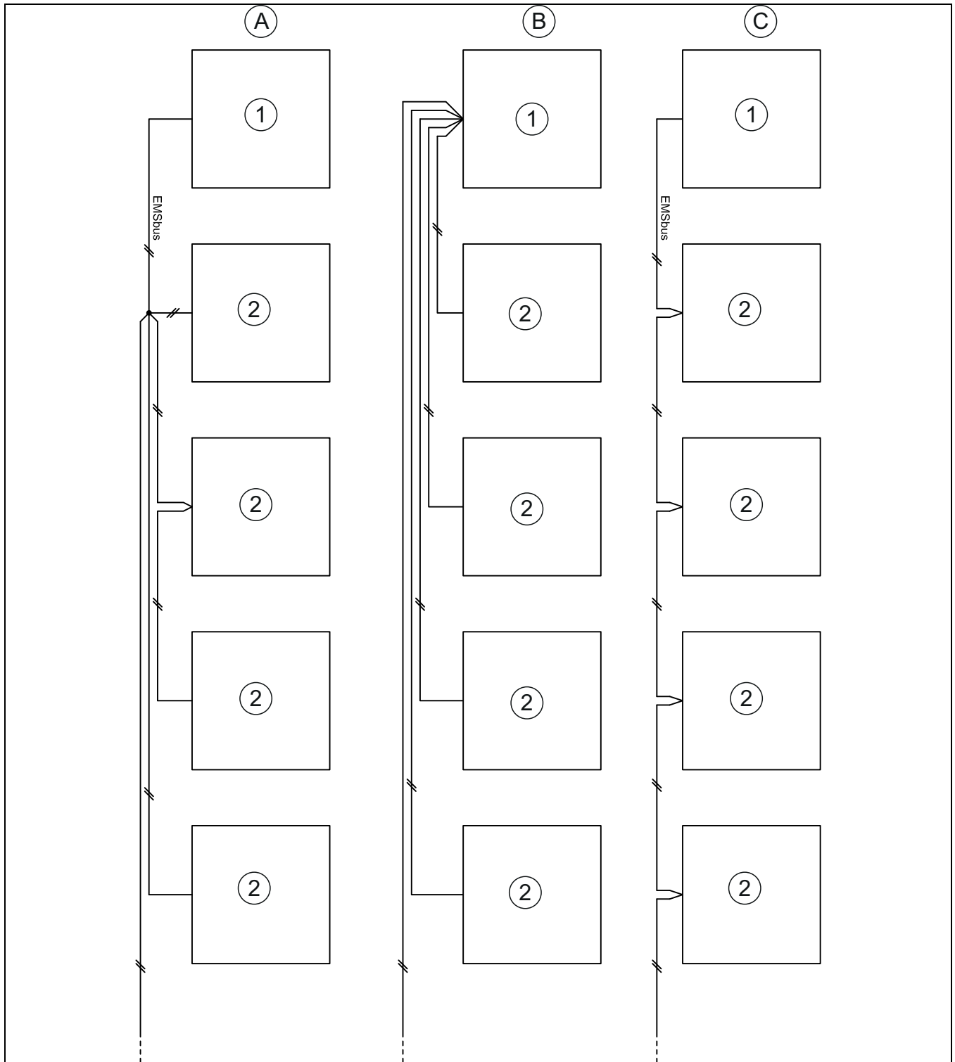
Fig. 46 Alternatives de raccordement pour bus EMS
