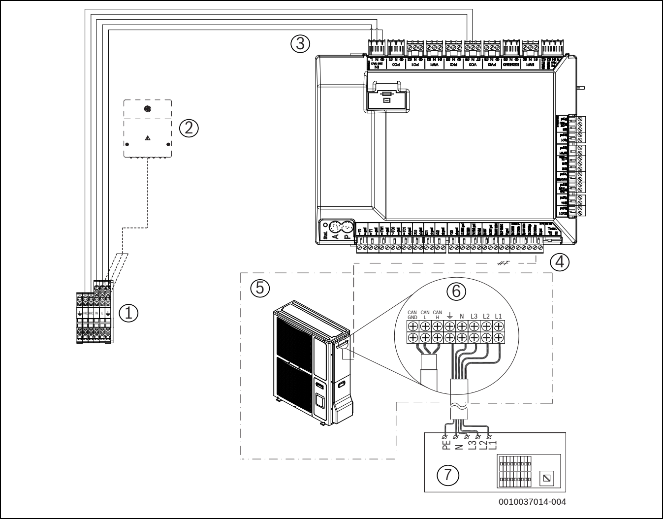
Fig. 45 Unité intérieure avec unité extérieure 400 V 3N ~
