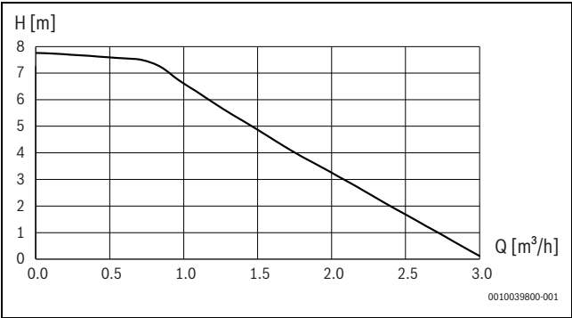
Fig. 32 Courbe caractéristique de capacité pour la pompe de circulation primaire (PC0)
