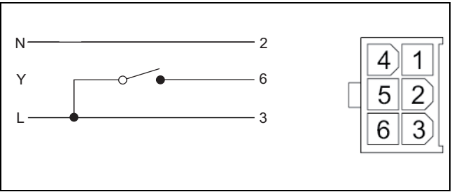
Fig. 23 Connecteur Molex
