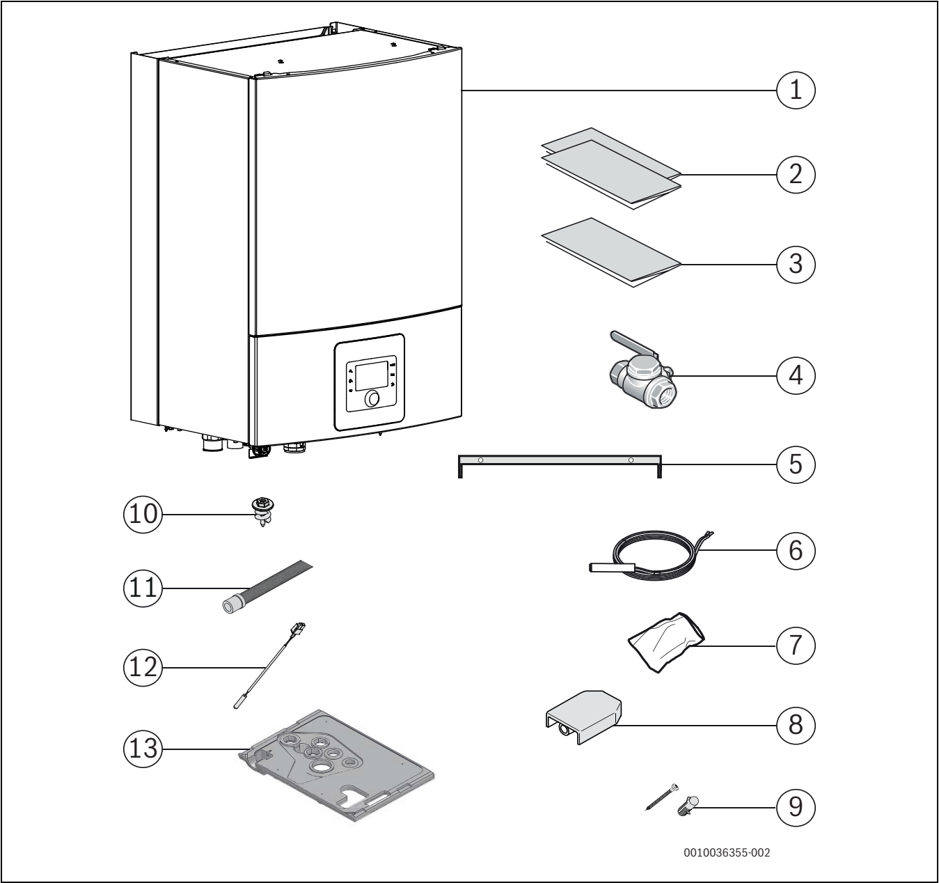
Fig. 2 Pièces fournies
