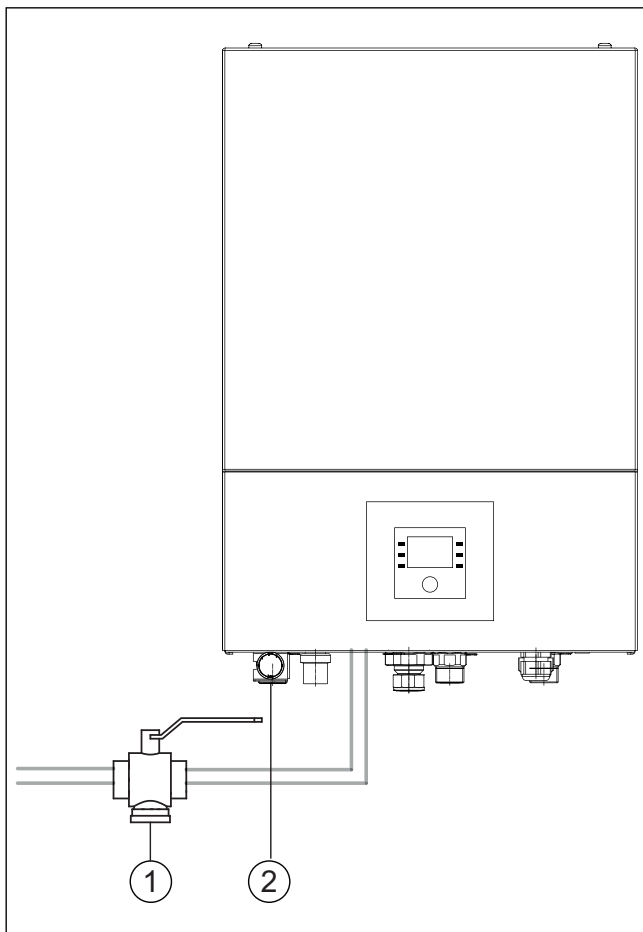
Fig. 6 Unité intérieure AWB
