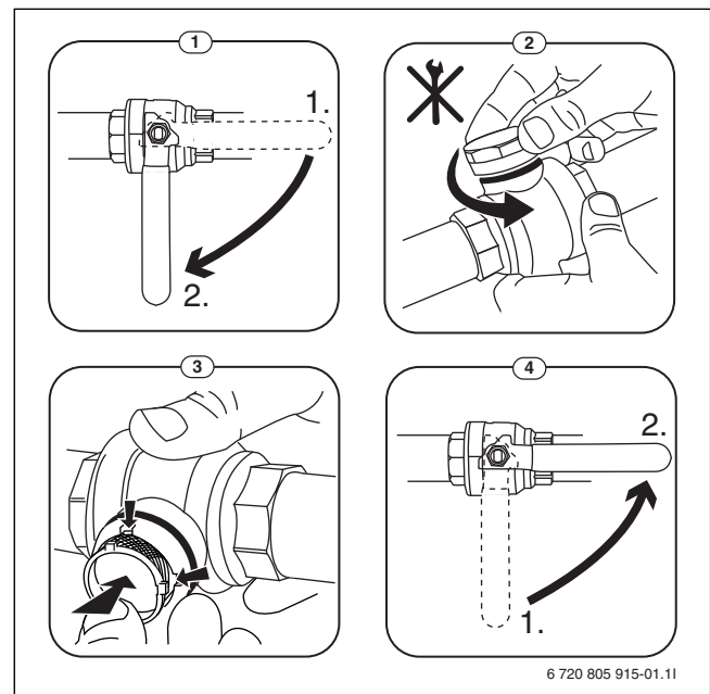
Fig. 7 Nettoyage du filtre
