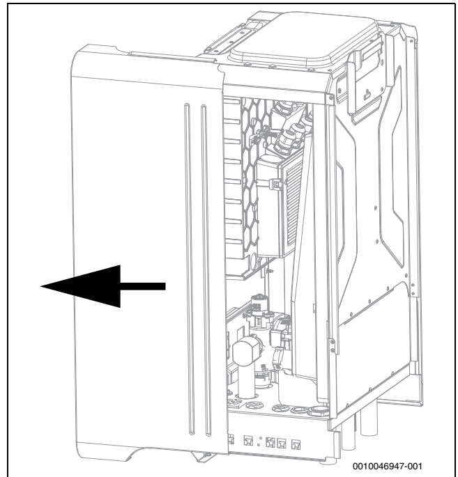
Bild 18 Seitenabdeckung abnehmen
