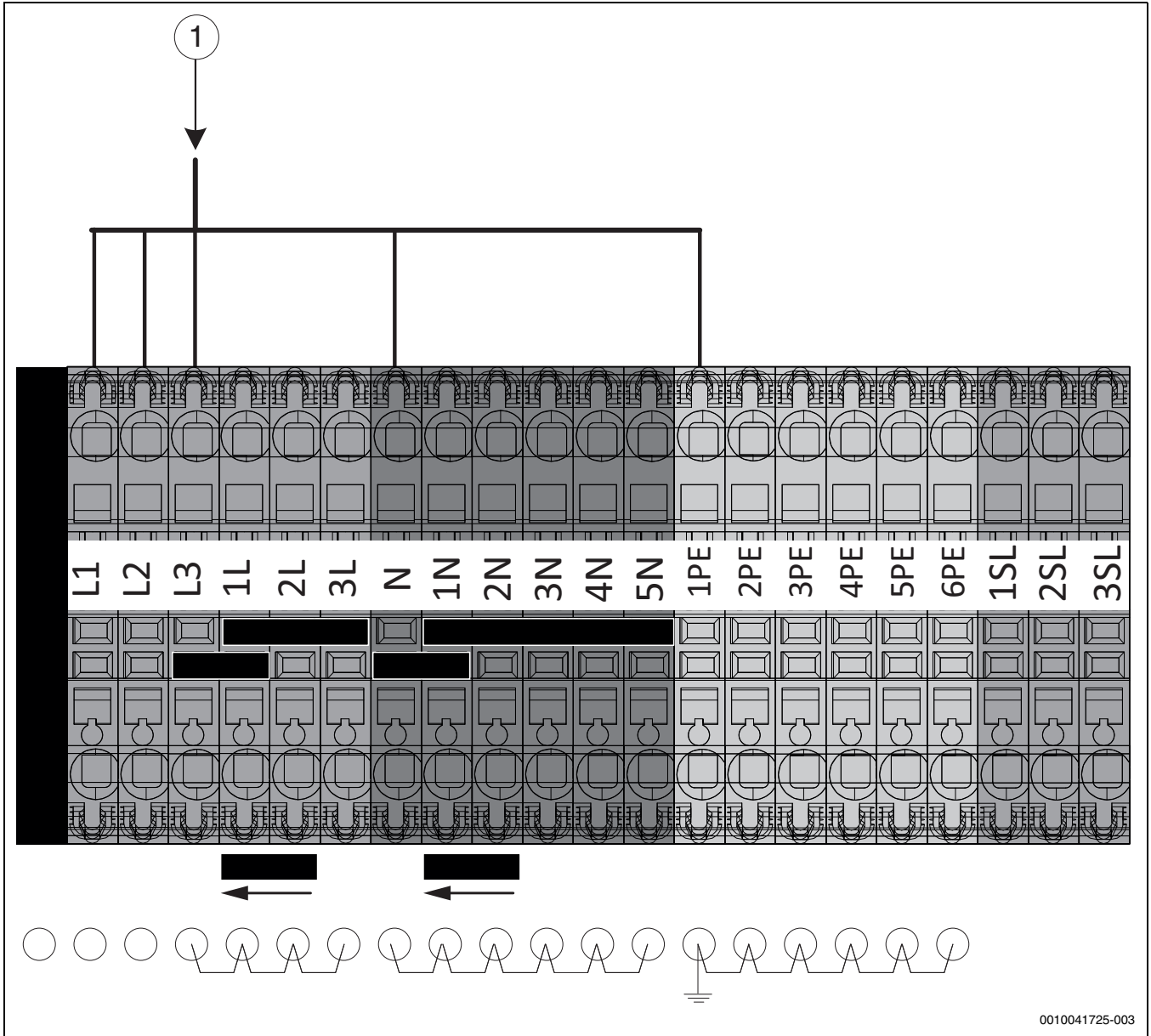
Bild 36 Elektrischer Anschluss
