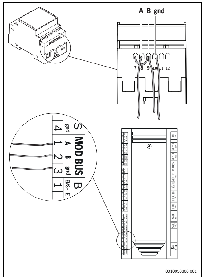
Bild 13 Power Meter 5000 an die Inneneinheit anschließen
