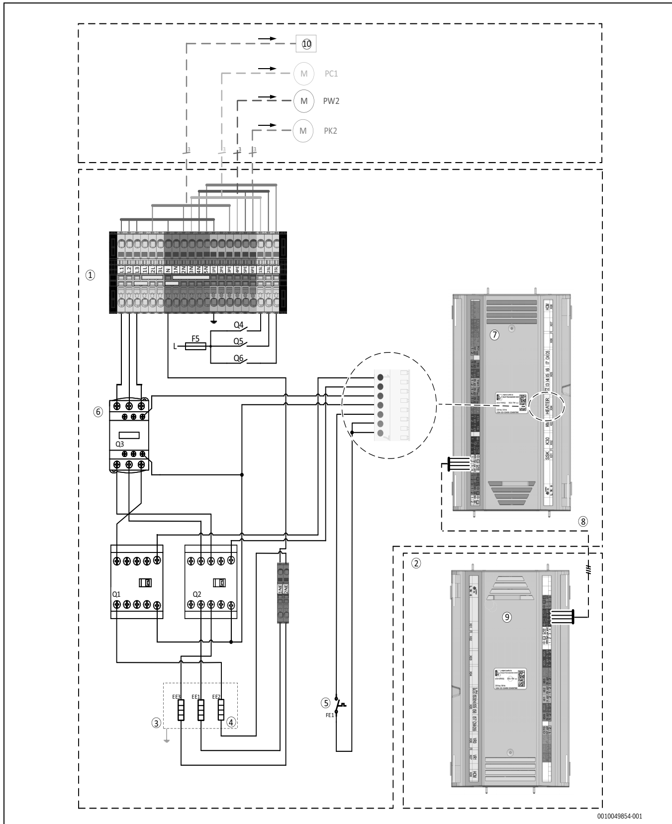
Bild 48 Spannungsversorgung Inneneinheit, Standard
