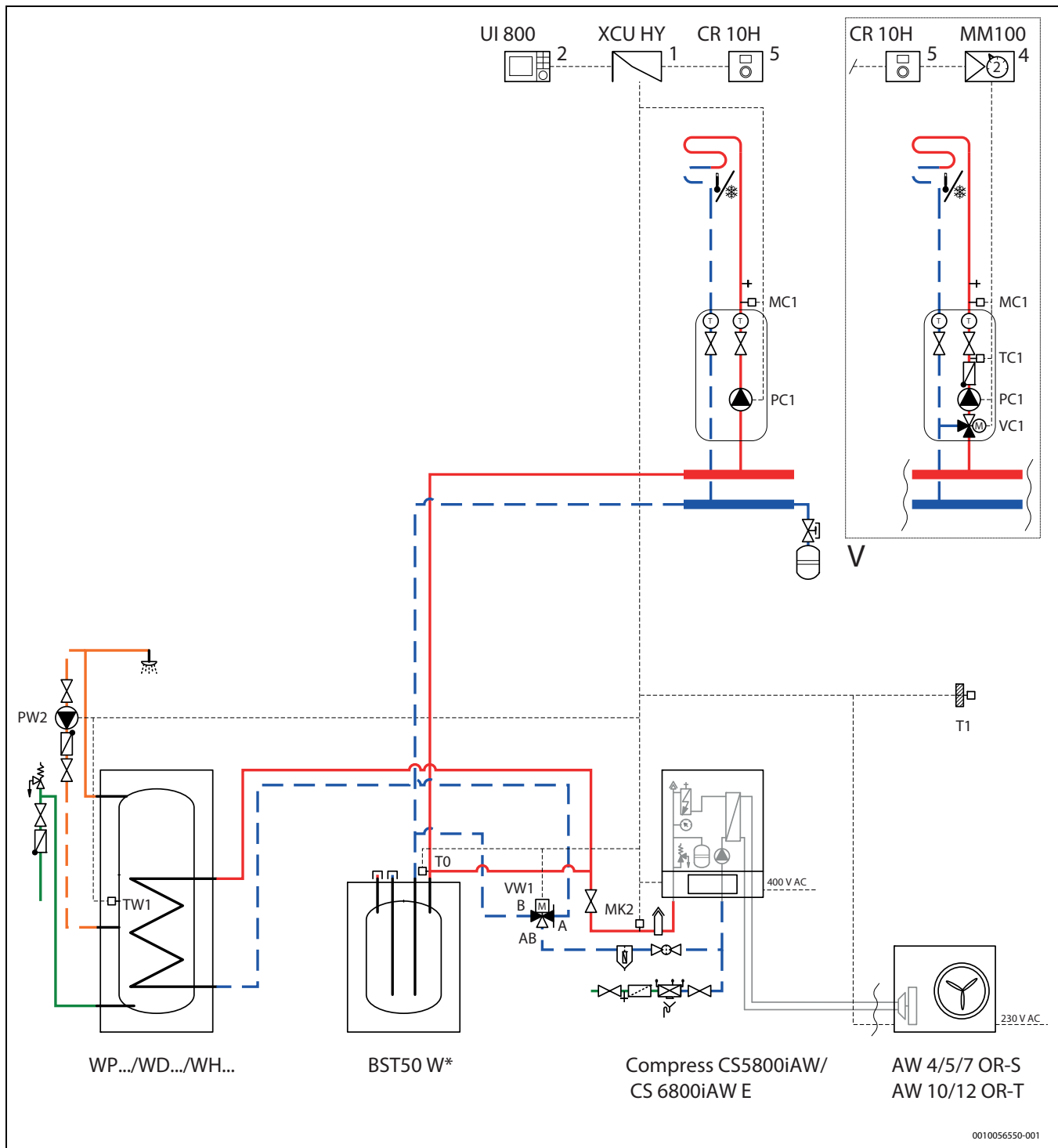
Bild 43 Wärmepumpe mit Inneneinheit, kleinem Pufferspeicher und Warmwasserbereiter
