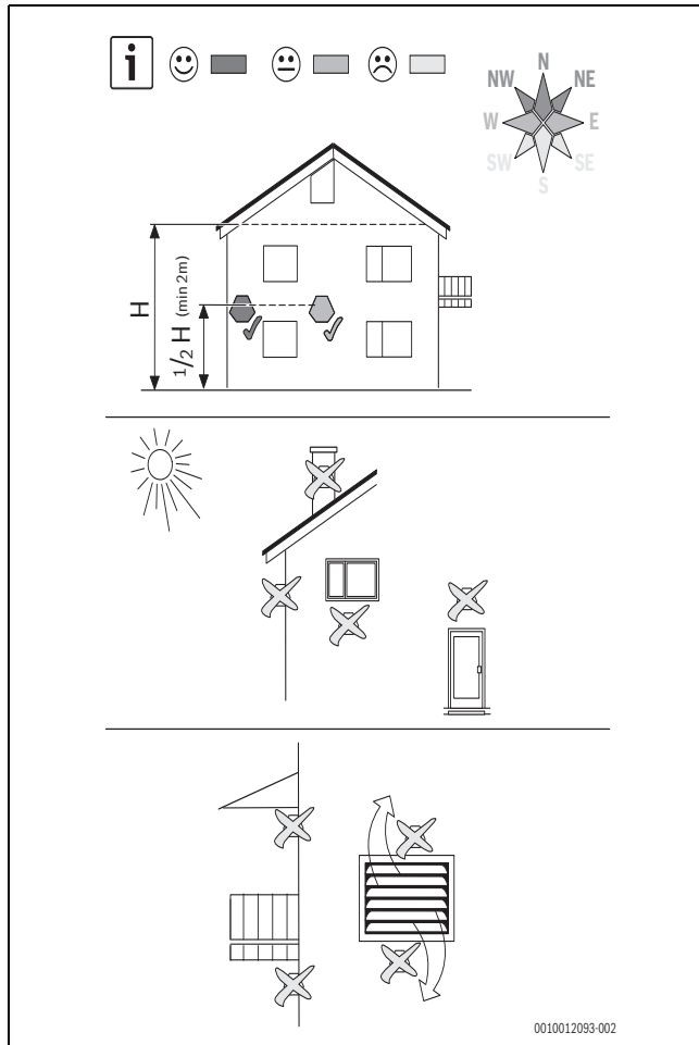
Bild 29 Position des Außentemperaturfühlers
