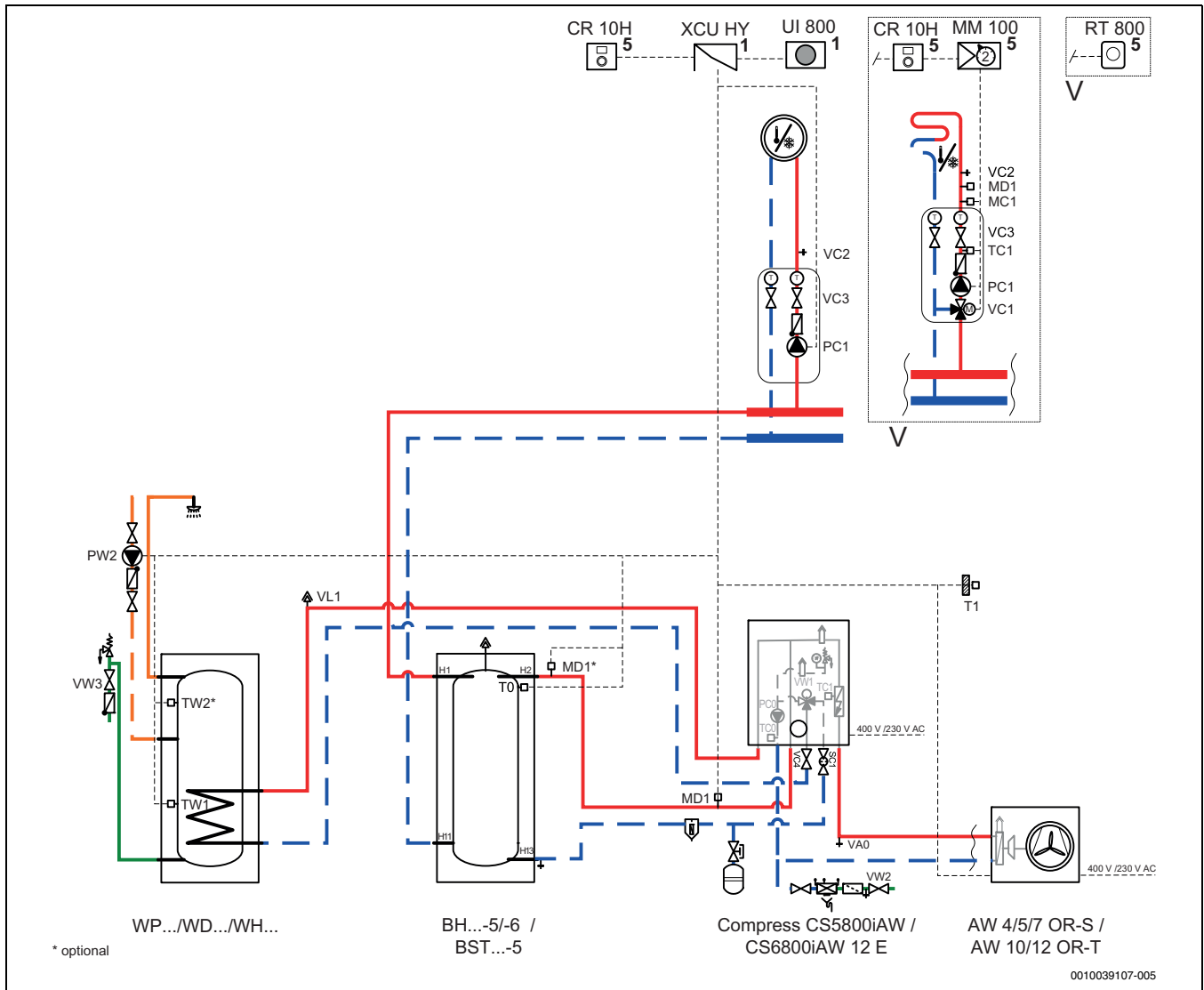
Bild 44 Wärmepumpe, Inneneinheit, Pufferspeicher und Warmwasserbereiter
