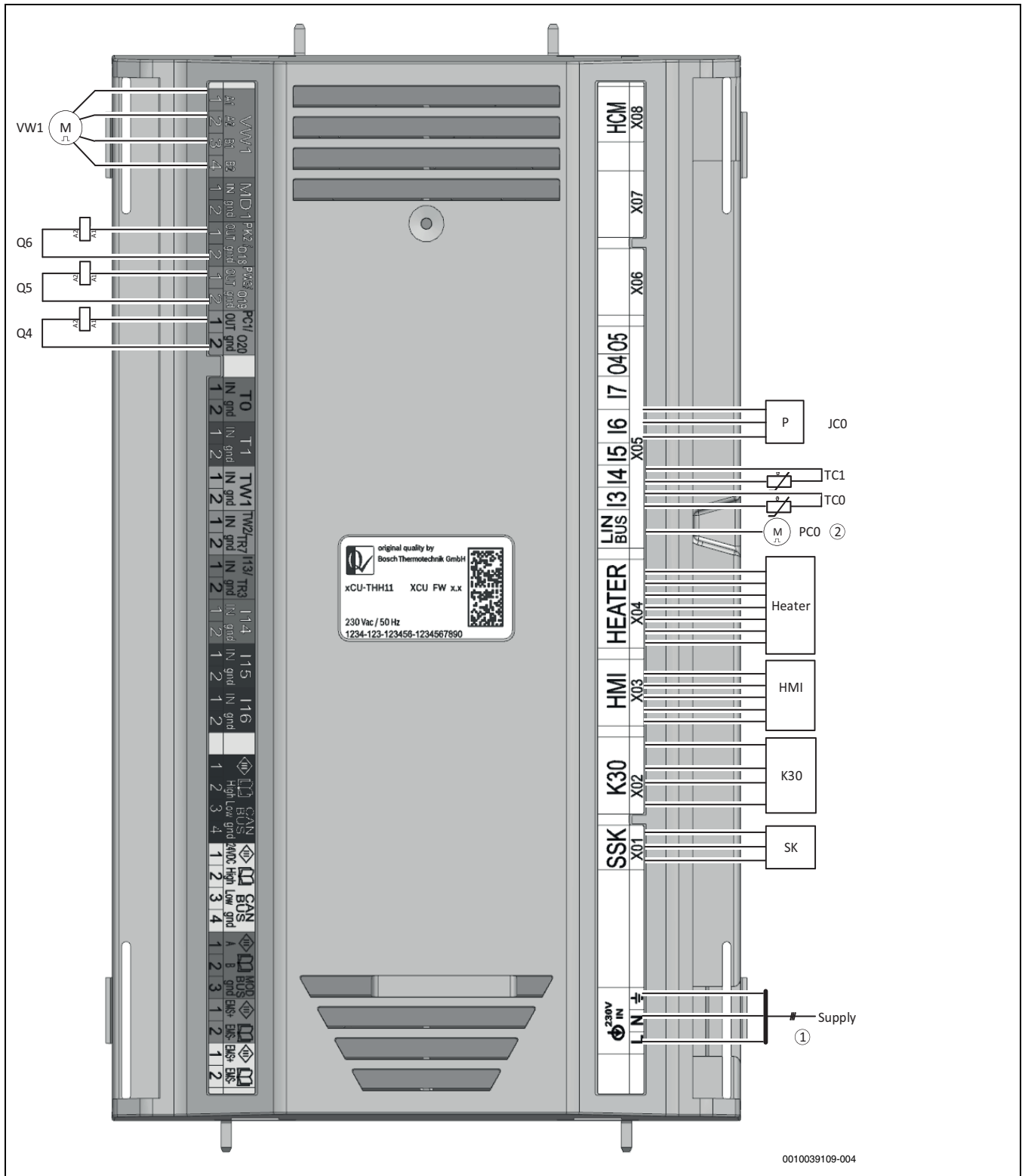
Bild 47 Schaltplan XCU-THH (XCU HY)
