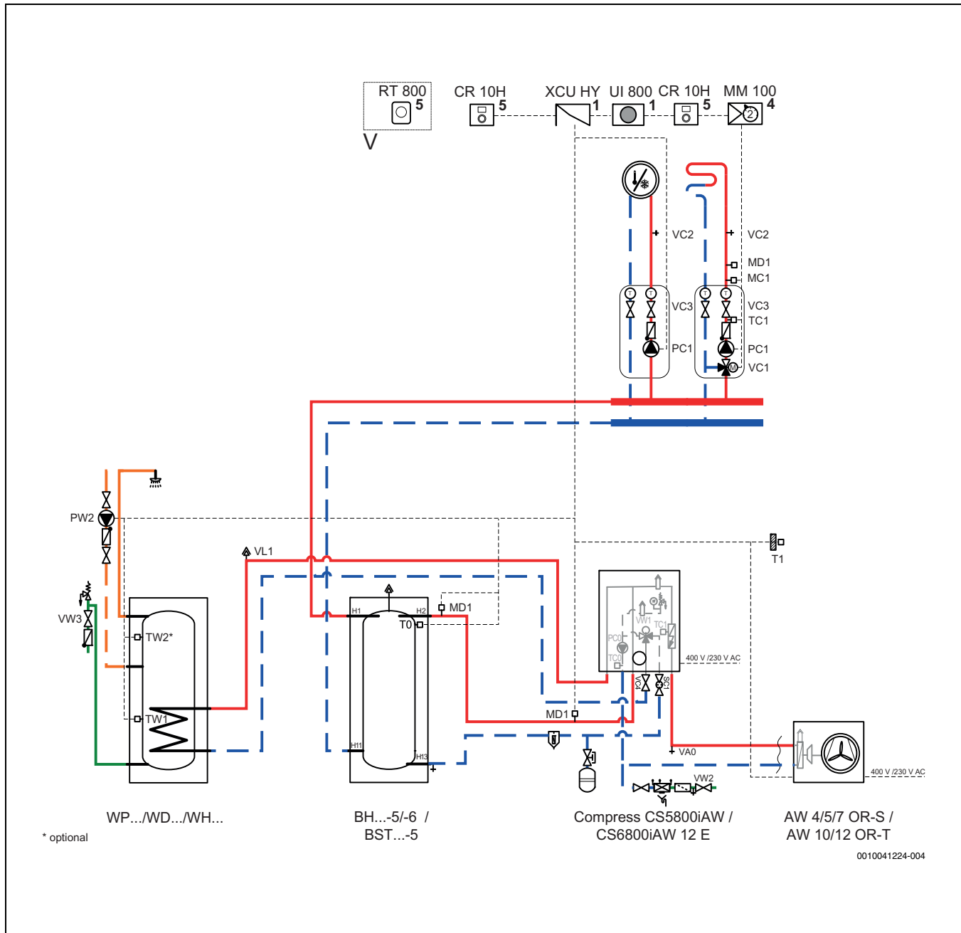
Bild 45 Wärmepumpe, zwei Heizkreise, Inneneinheit, Pufferspeicher und Warmwasserspeicher
