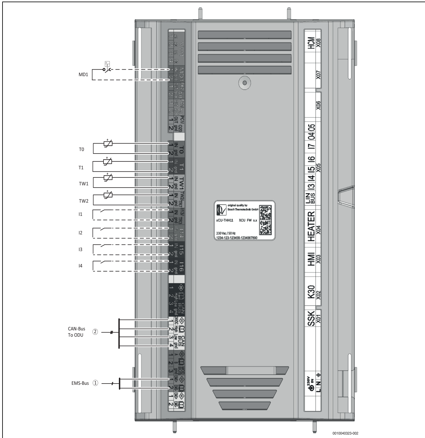
Bild 39 Anschlüsse
