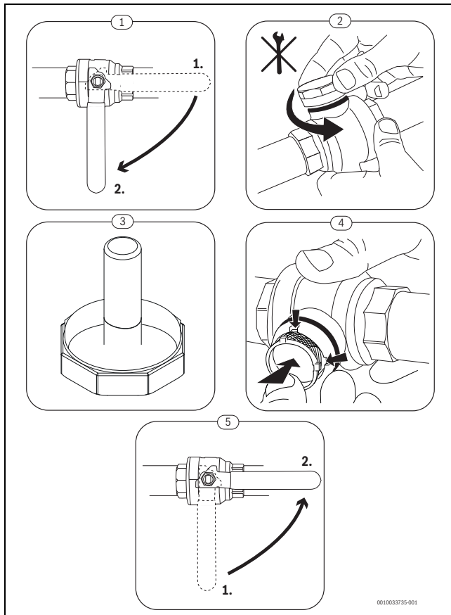
Bild 42 Siebreinigung
