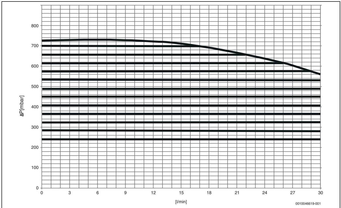
Bild 46 Leistungsdiagramm für Pumpe PC0
