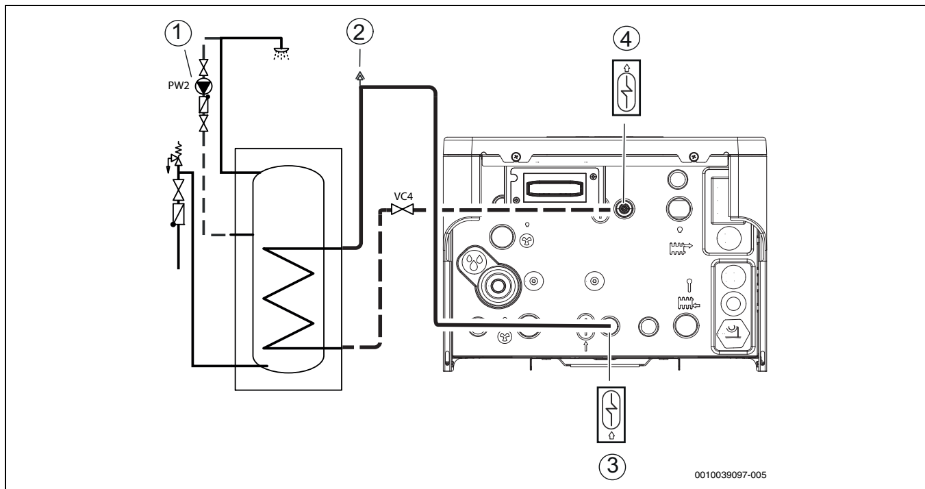
Bild 23 Trinkwasseranschlüsse Inneneinheit
