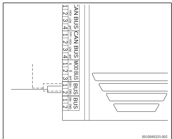
Bild 28 EMS-Anschluss
