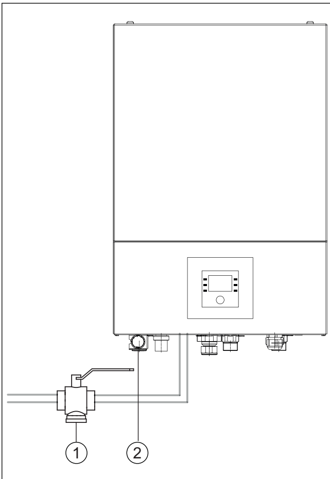
Afb. 6 Binneneenheid AWB
