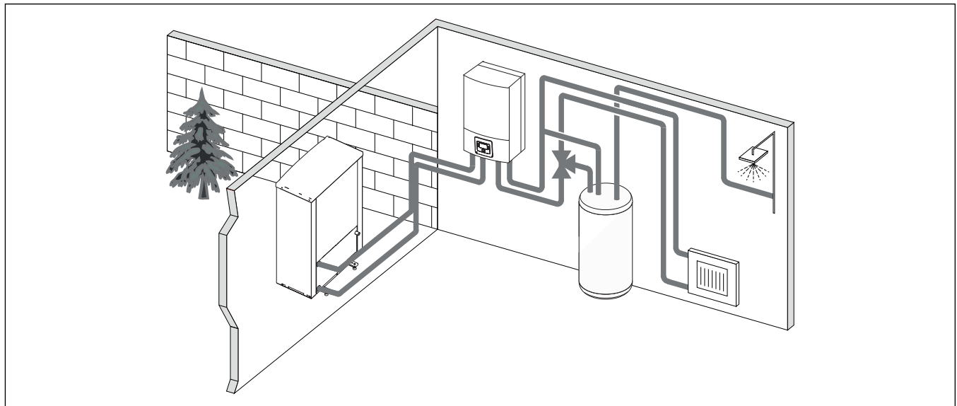
Afb. 3 Warmtepomp Compress 6000 AW, binneneenheid AWE met elektrische bijverwarming en externe warmwaterboiler
