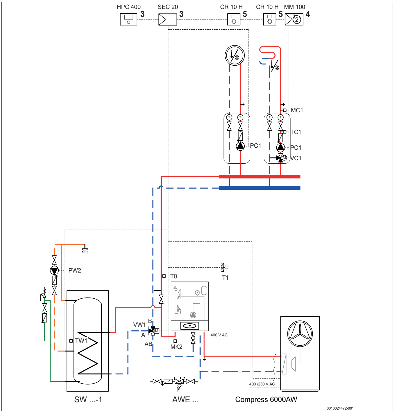
Fig. 25 Chauffage d'appoint électrique avec préparateur d'eau chaude sanitaire
