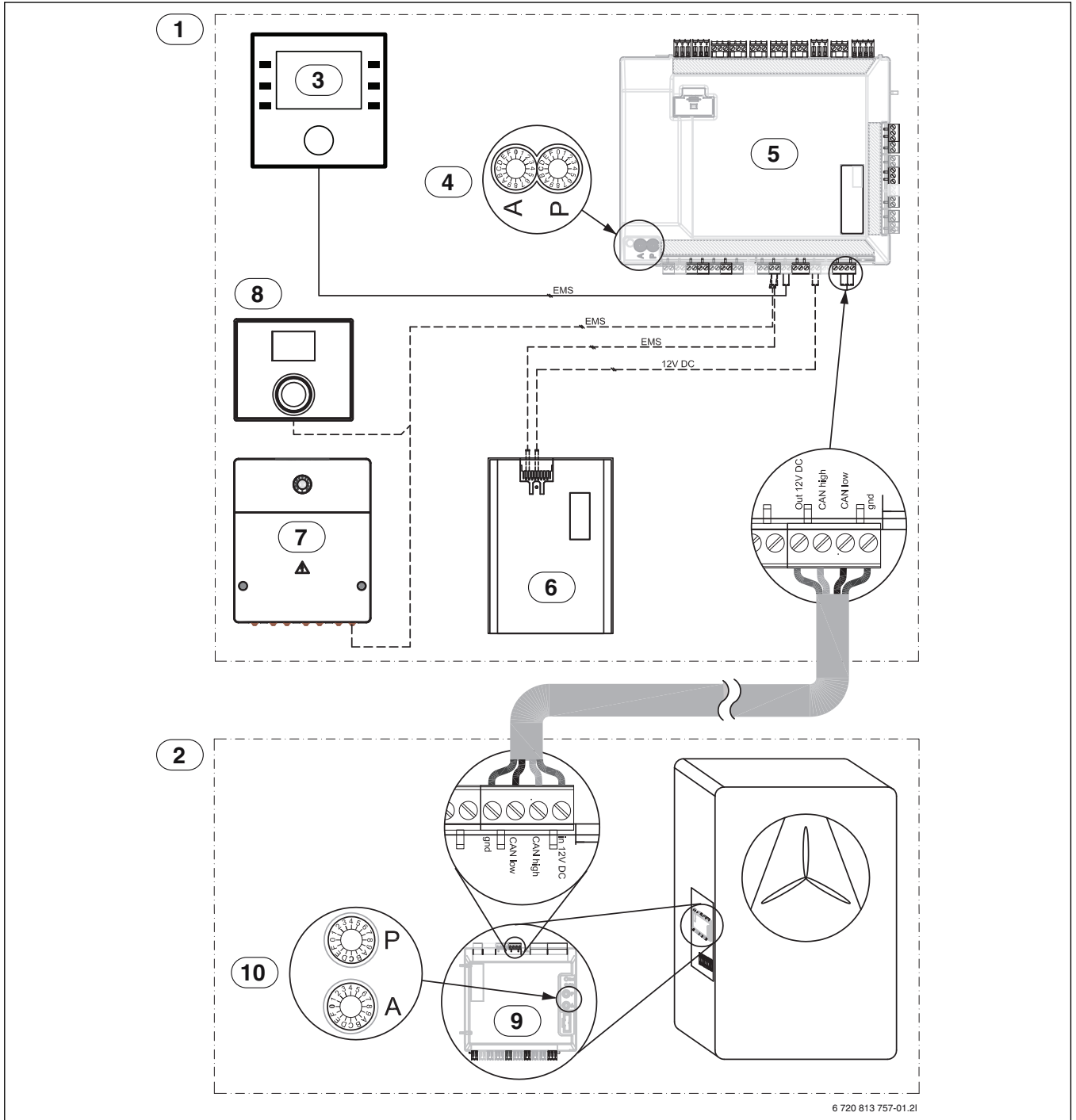
Fig. 26 CAN-BUS/EMS-BUS pour unité intérieure avec chauffage d'appoint électrique – aperçu
