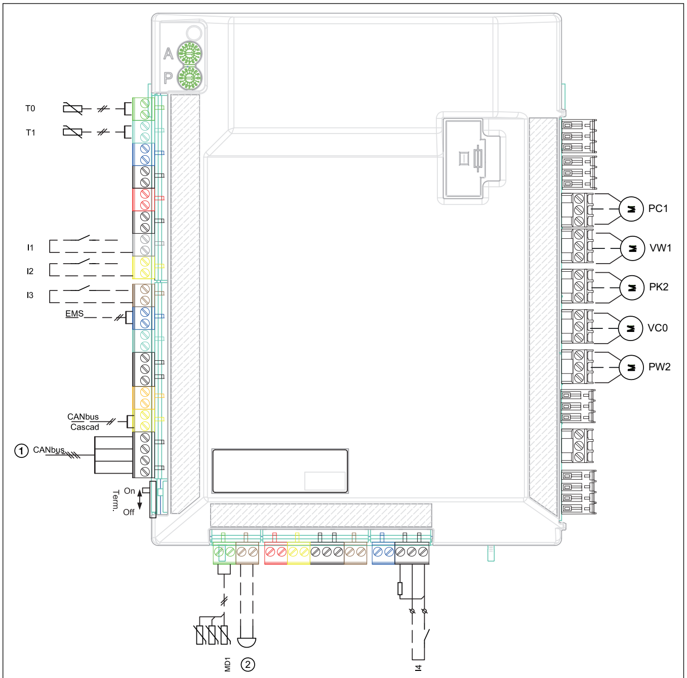
Fig. 11 Raccordements du module d'installation
