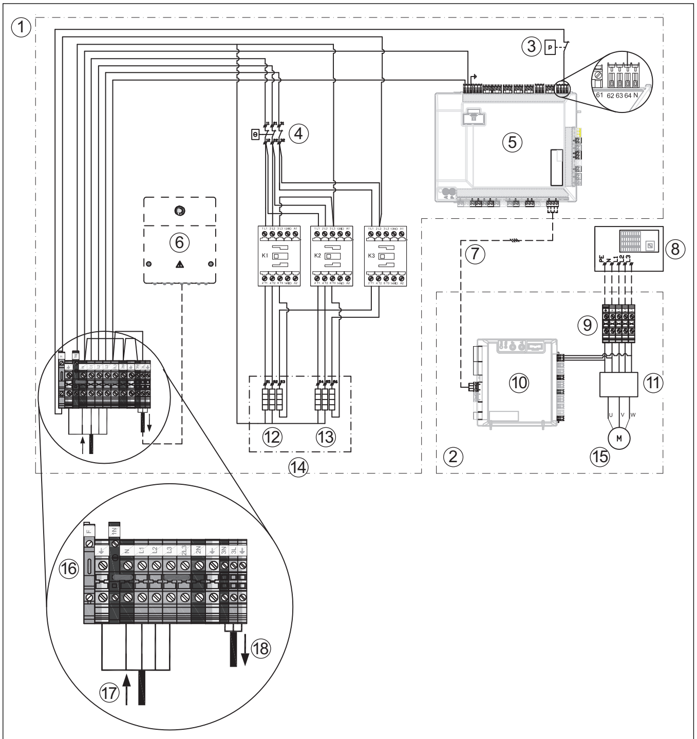
Fig. 28 Pompe à chaleur (courant triphasé) avec chauffage d'appoint électrique intégré (courant triphasé)
