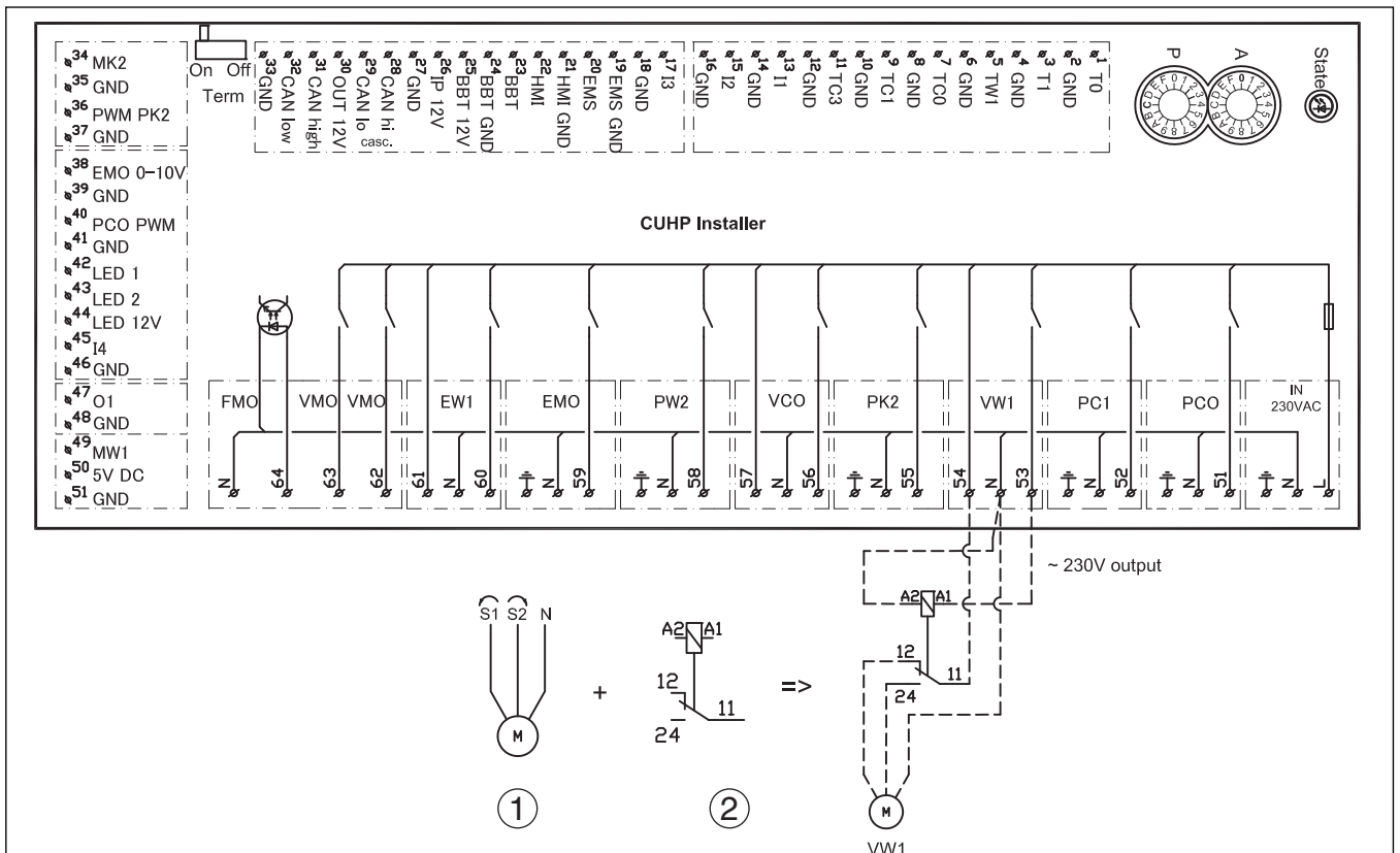
Fig. 30 Alternative d'installation de la vanne sélective
