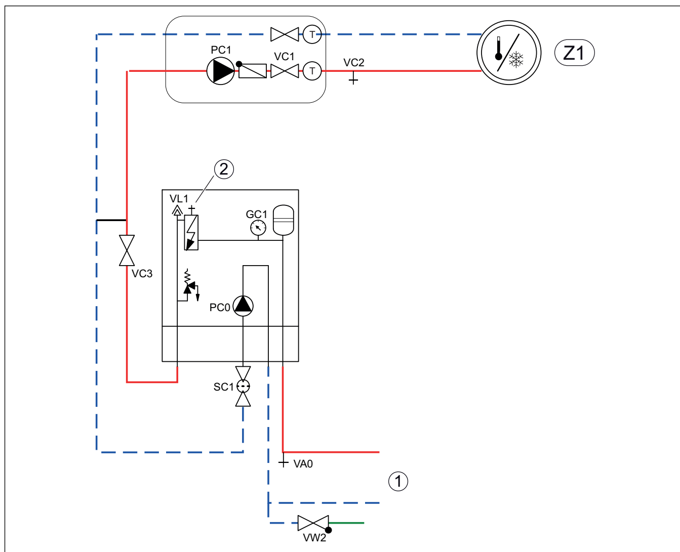
Fig. 6 Unité intérieure avec chauffage d'appoint électrique intégré et système de chauffage
