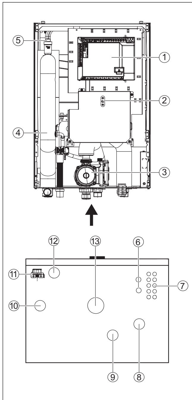
Fig. 2 Composants et raccords de l'unité intérieure avec chauffage auxiliaire
