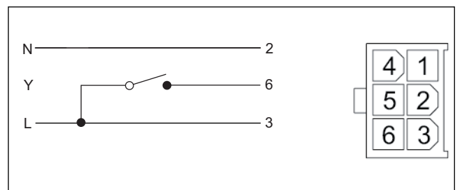
Fig. 20 Connecteur Molex
