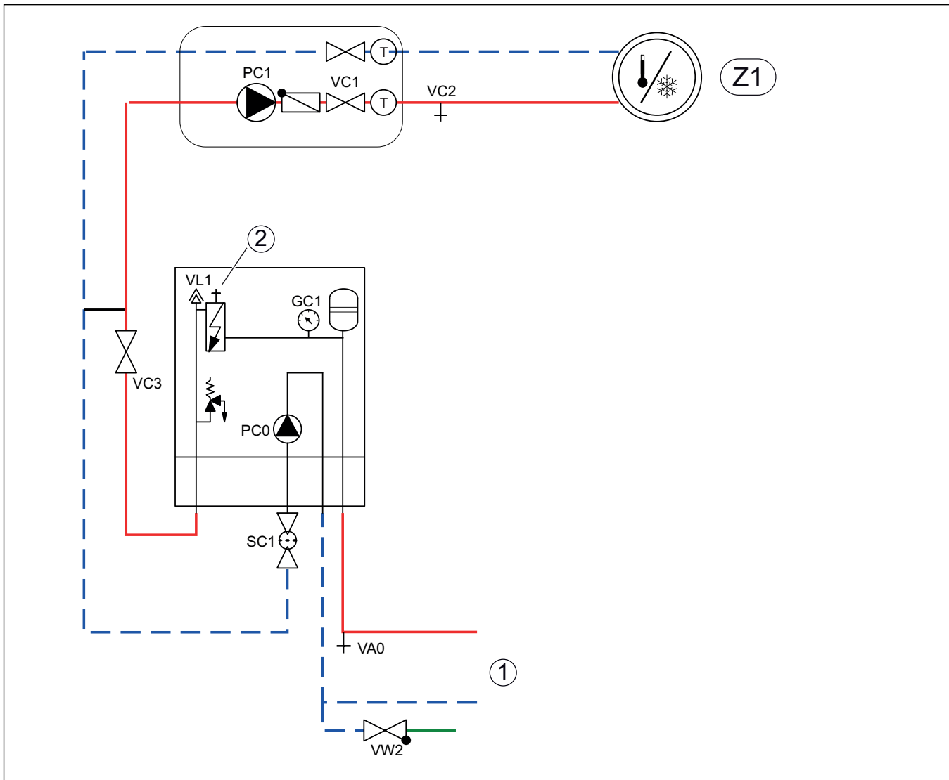
Fig. 13 Unité intérieure avec chauffage d'appoint électrique intégré et système de chauffage
