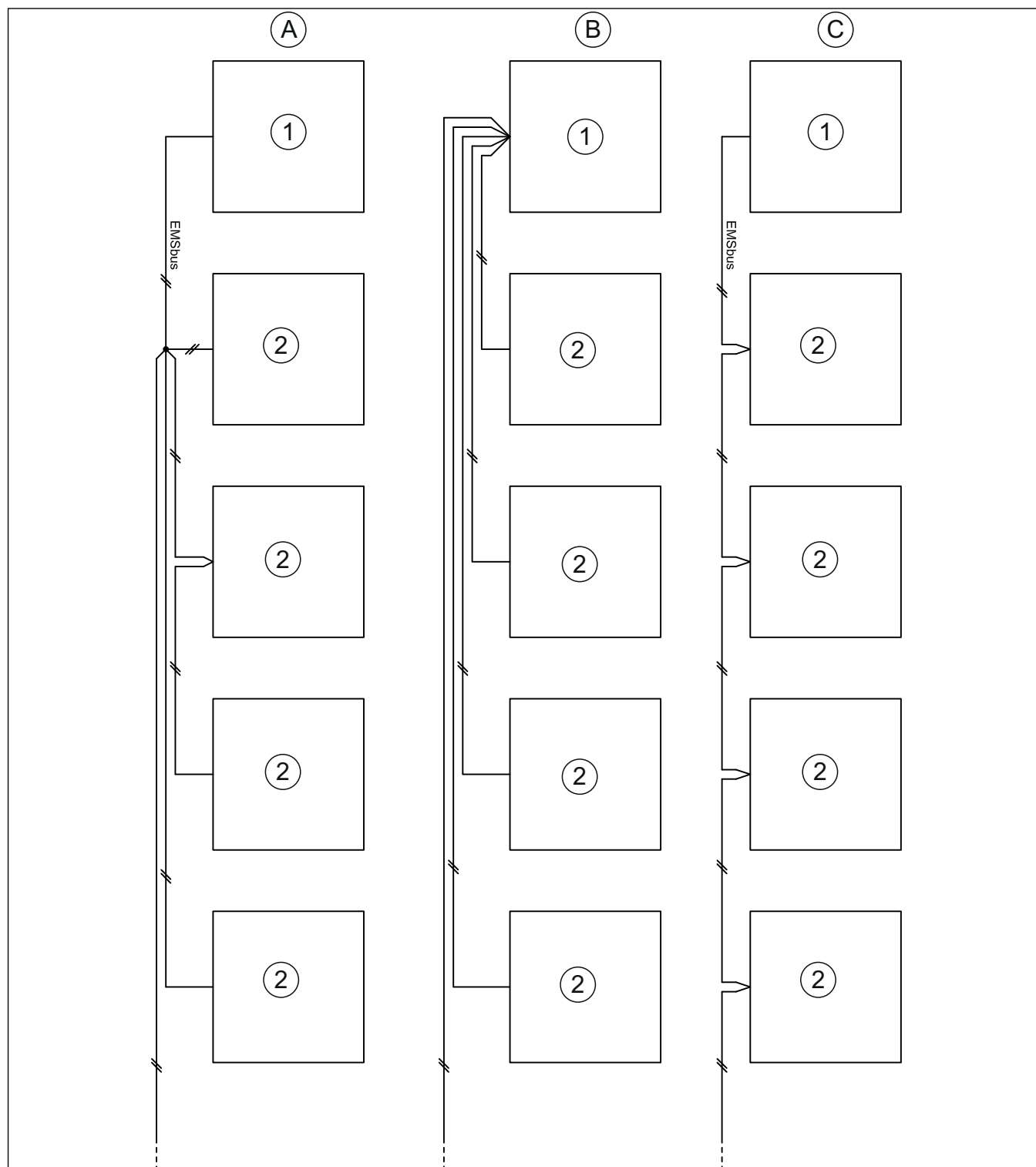
Fig. 12 Alternatives de raccordement pour bus EMS
