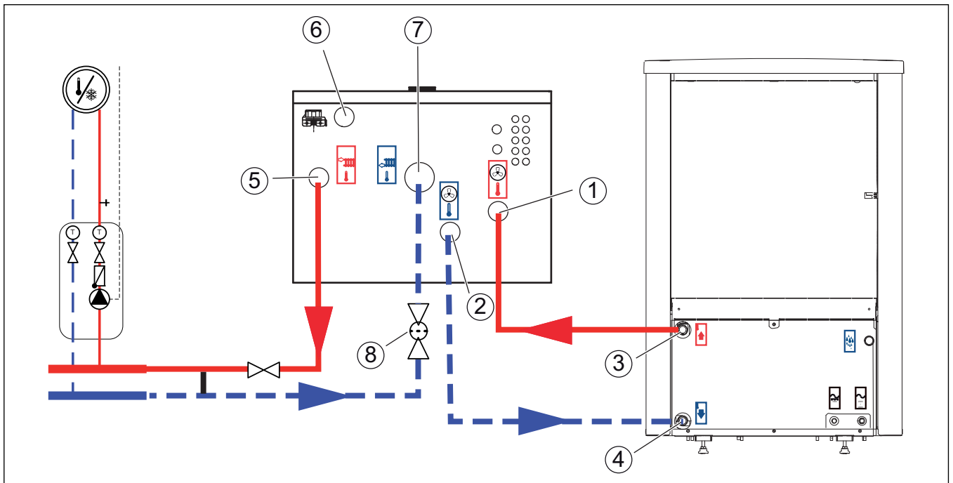
Fig. 5 Raccordement de l'unité intérieure avec chauffage d'appoint électrique à la pompe à chaleur et l'installation de chauffage
