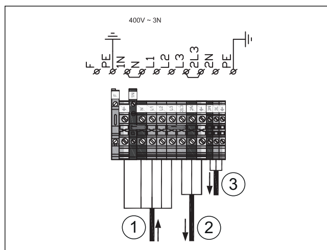
Fig. 10 Raccordement électrique standard en cas de chauffage d'appoint électrique intégré
