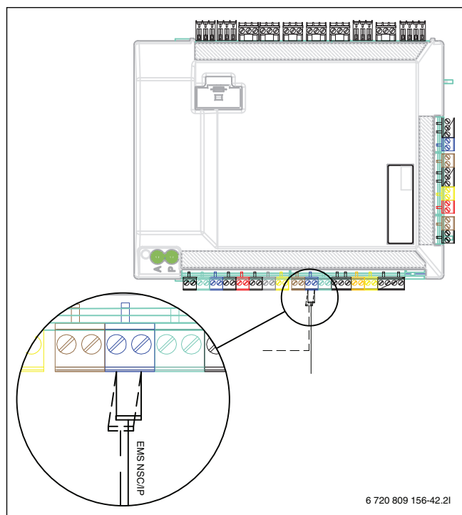
Fig. 15 Raccordement EMS sur le module d'installation
