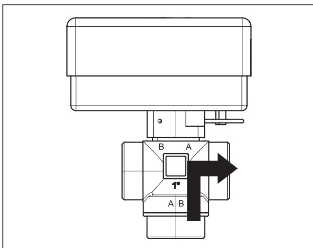
Fig. 18 Contact fermé, raccordement A ouvert
