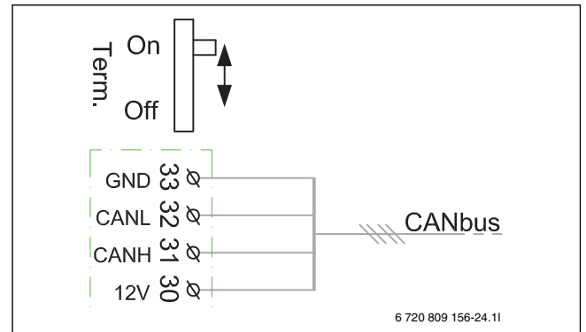
Fig. 7 Terminaison CAN-BUS
