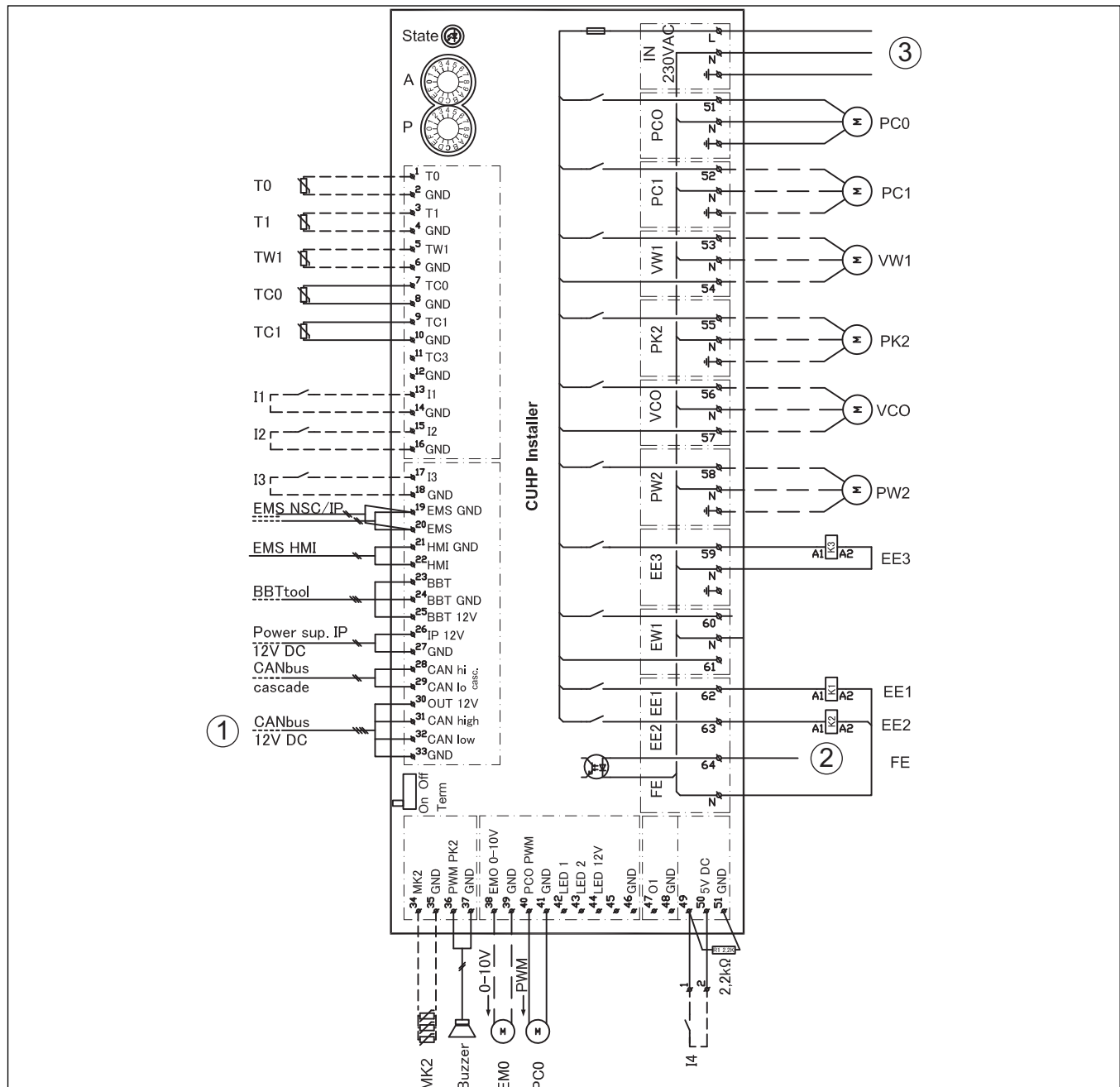
Fig. 29 Schéma de connexion du module d'installation avec chauffage d'appoint électrique intégré
