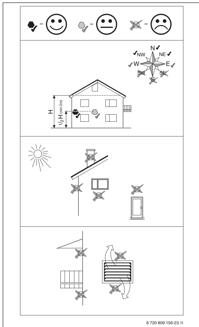
Fig. 8 Placement de la sonde de température extérieure
