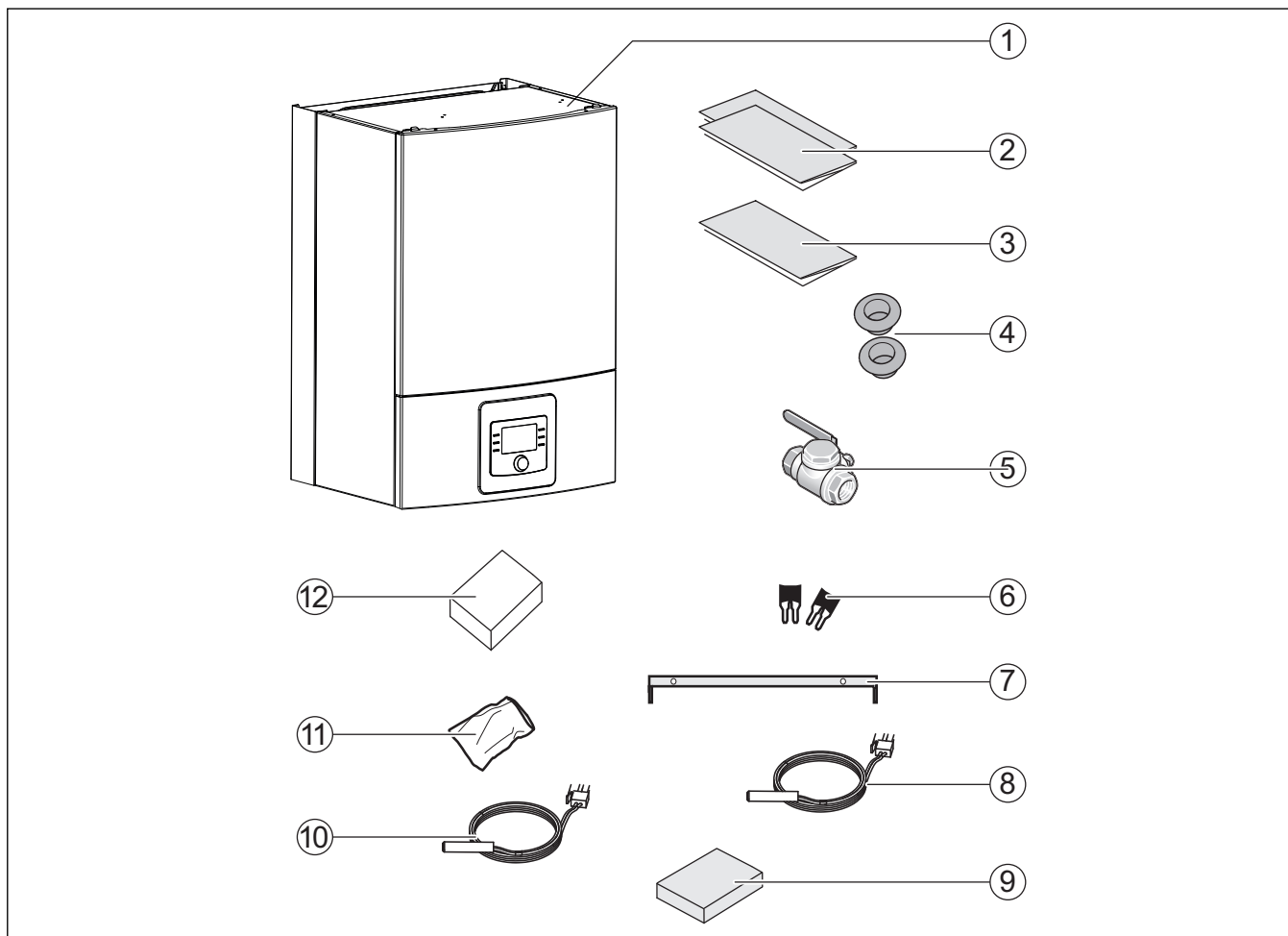
Fig. 1 Contenu de livraison
