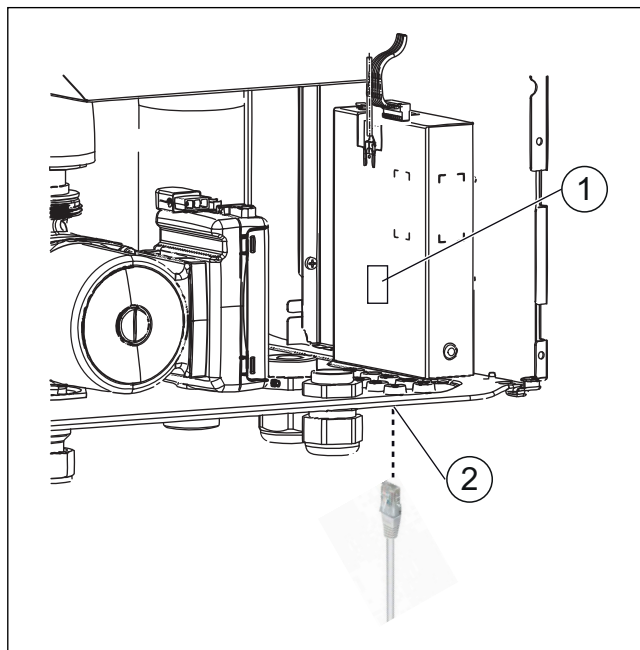
Fig. 22 Module IP
