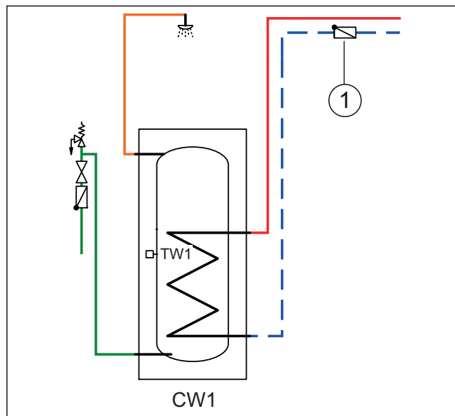
Fig. 16 Ballon d'eau chaude sanitaire
