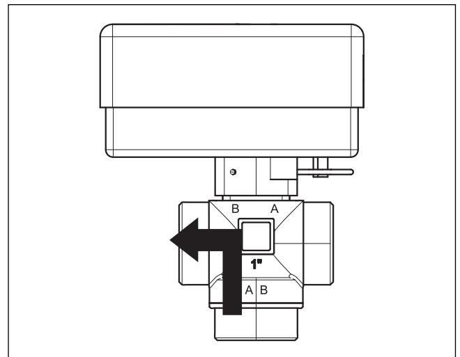
Fig. 19 Contact ouvert, raccordement B ouvert
