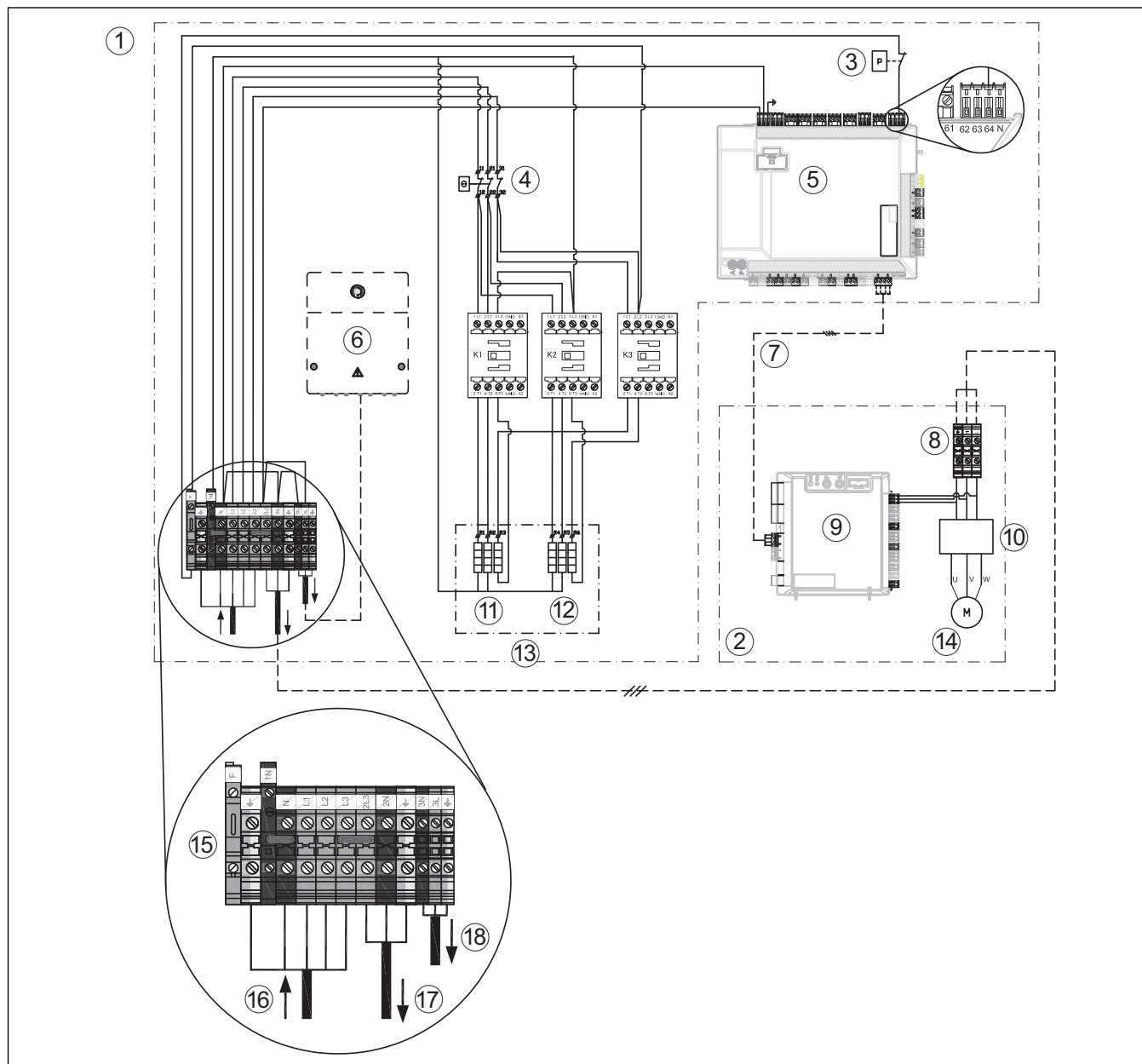
Fig. 27 Pompe à chaleur monophasée avec chauffage d'appoint électrique intégré (courant triphasé)
