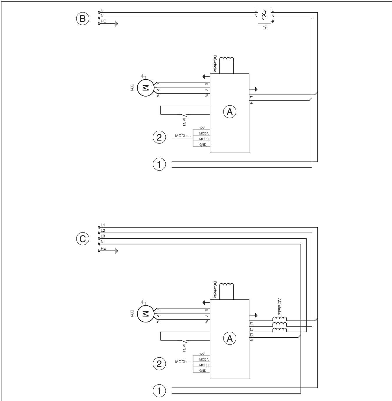
Fig. 22 Schéma de connexion pour convertisseur, courant alternatif/courant triphasé
