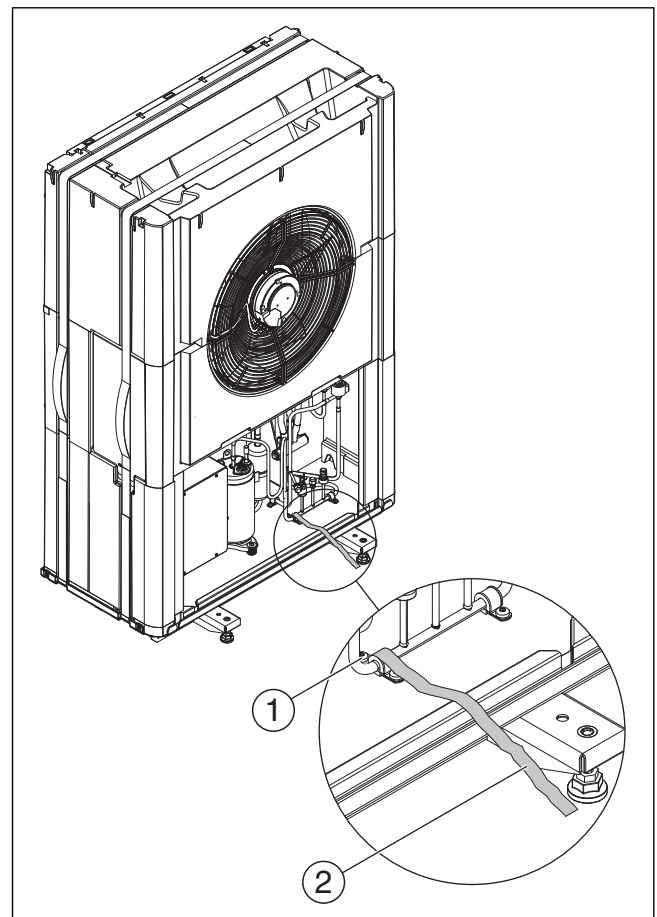
Fig. 12 Sécurisation pour le transport
