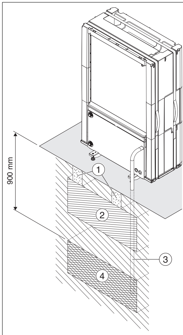
Fig. 11 Evacuation des condensats dans un lit de gravier
