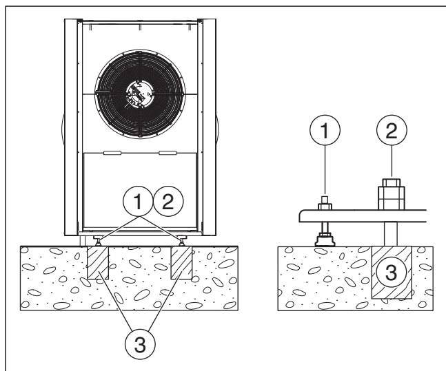
Fig. 13 Fixation de la pompe à chaleur
