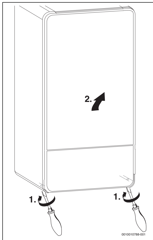
Fig. 23 Retirer l'habillage
