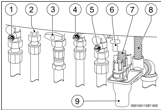
Fig. 28 Raccords côté gaz et eau (accessoires)
