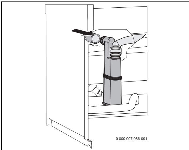
Fig. 25 Monter le tuyau sur le siphon des condensats
