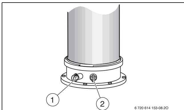
Fig. 48 Buse de mesure des fumées et de l'air de combustion
