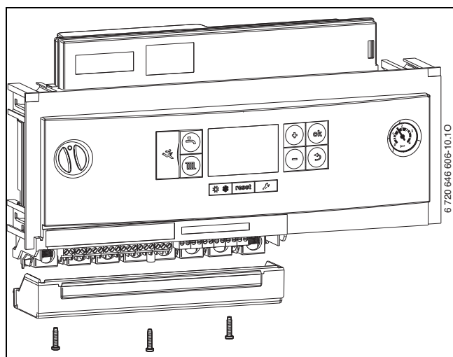
Fig. 72 Retirer le cache
