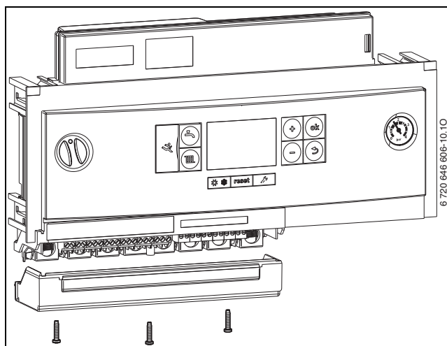
Fig. 30 Retrait du revêtement
