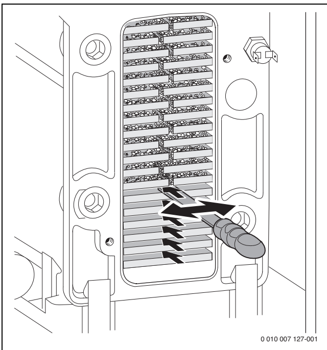
Fig. 54 lame de nettoyage
