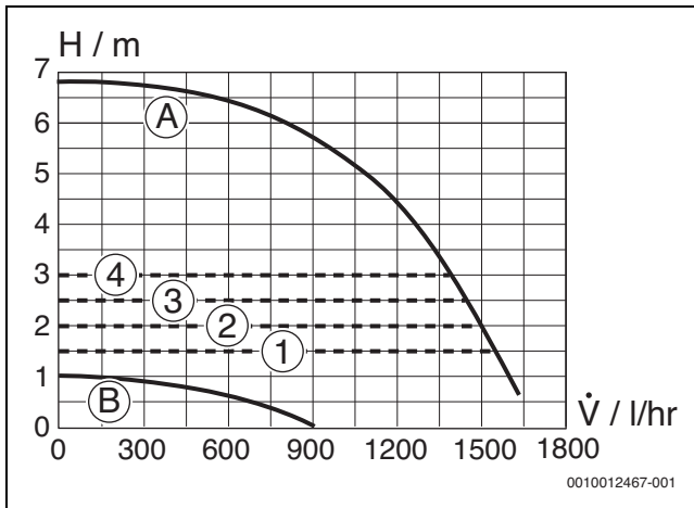
Fig. 80 Diagrammes de pompe et courbes caractéristiques de pompe
