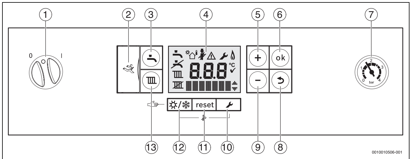
Fig. 32 Tableau de commande avec cache ouvert
