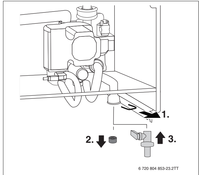
Fig. 26 Monter le robinet de remplissage et de vidange
