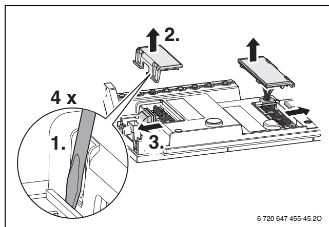
Fig. 74 Retirer le cache
