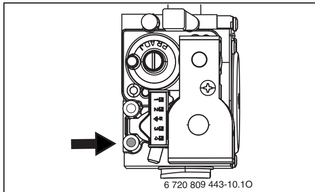
Fig. 46 Tubulures de mesure pour la pression de raccordement du gaz
