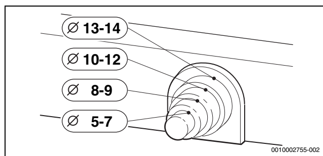
Fig. 31 Adaptation du serre-câbles au diamètre du câble
