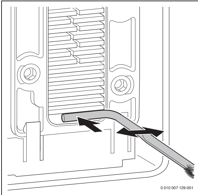
Fig. 57 Nettoyer le réservoir à condensats
