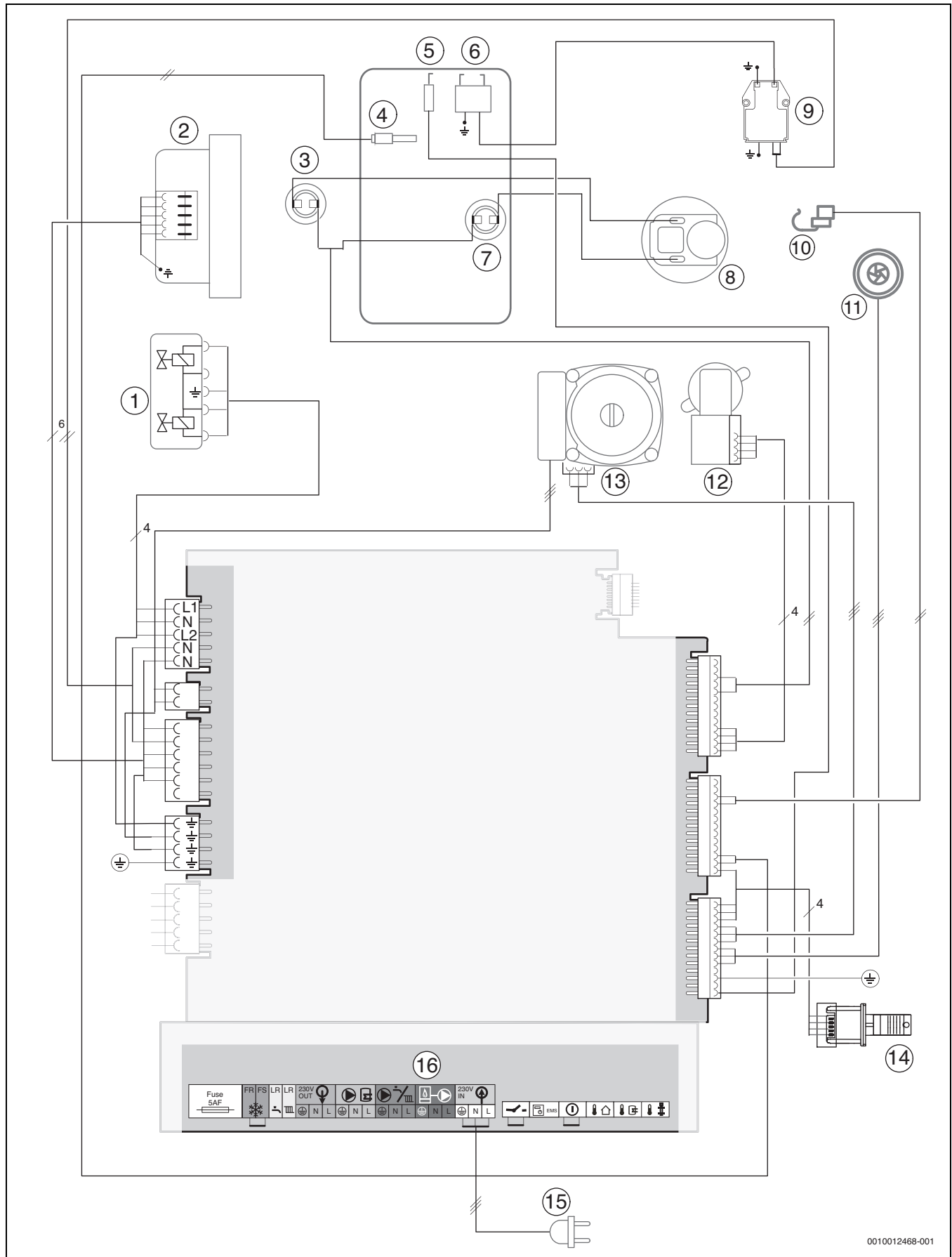
Fig. 78 Câblage électrique
