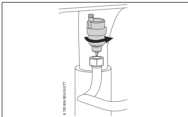
Fig. 64 Démontez le purgeur automatique
