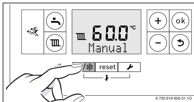
Fig. 43 Régler le mode manuel
