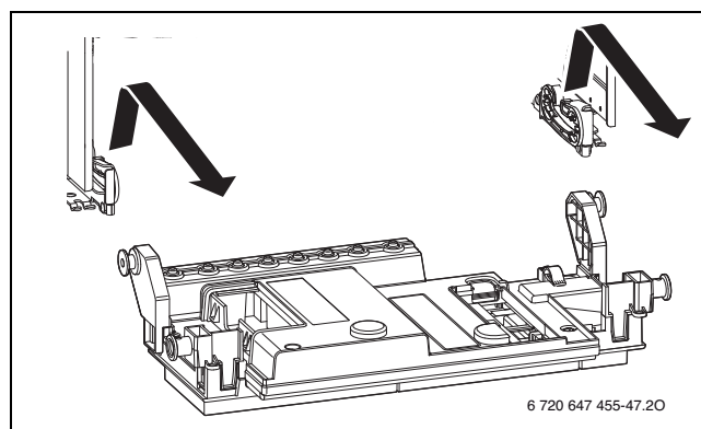
Fig. 75 Déclipser l'appareil de commande
