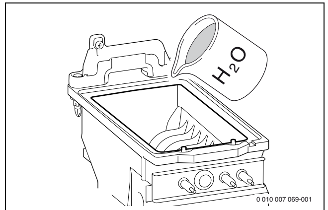
Fig. 56 Purge
