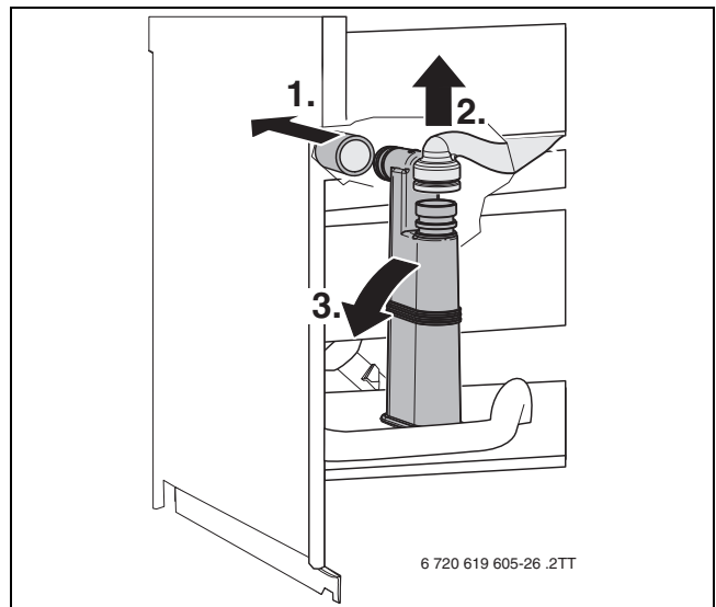
Fig. 58 Démontez le siphon des condensats
