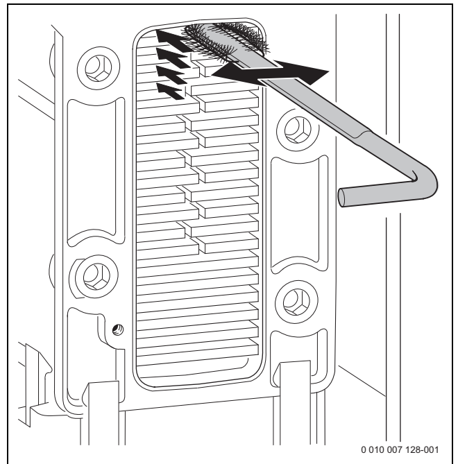
Fig. 55 Nettoyer le corps de chauffe à l'aide de la brosse
