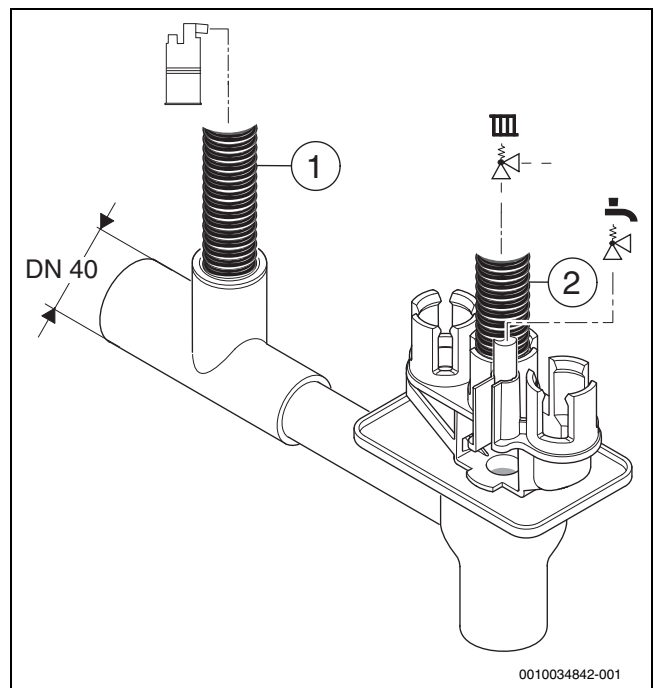
Fig. 27 Monter le tuyau des condensats et le tube de la soupape de sécurité sur le siphon
