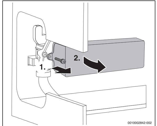
Fig. 61 Démontage de l'échangeur à plaques
