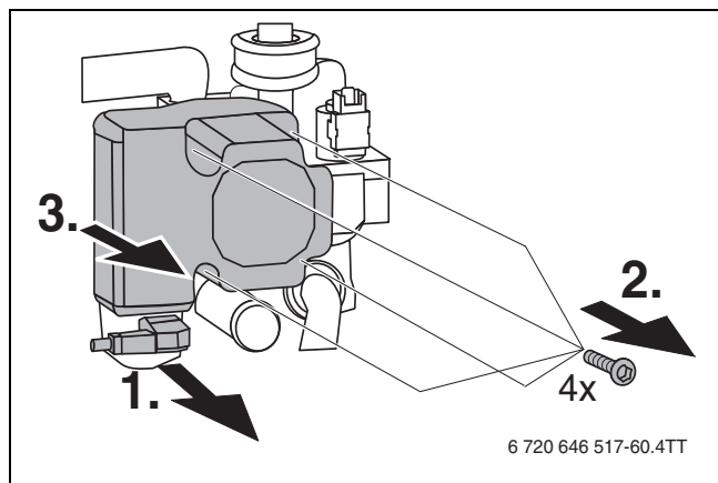
Fig. 71 Démontez la pompe de chauffage
