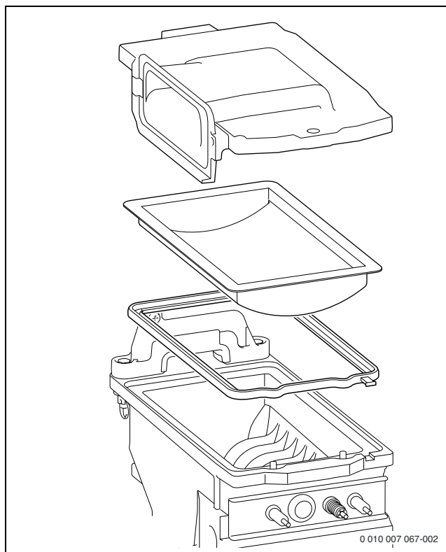
Fig. 52 Brûleur
