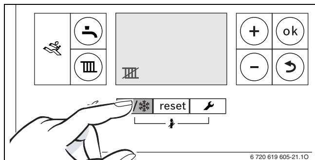
Fig. 41 Mettre en marche le mode été manuel
