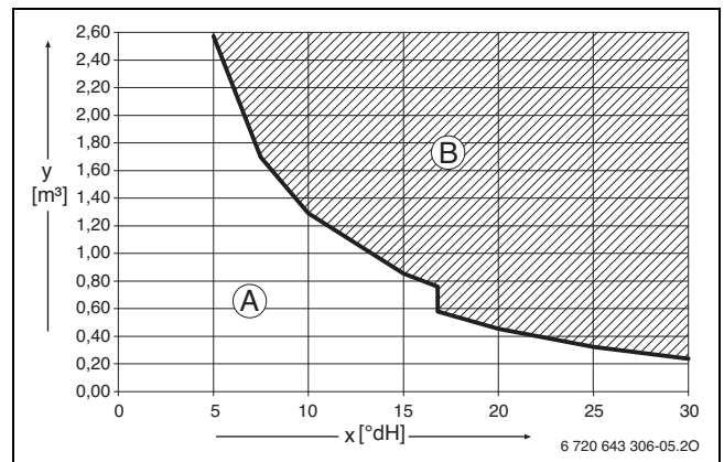
Fig. 20 Conditions requises pour l'eau de remplissage et d'appoint en °dH sur les appareils < 50 kW
