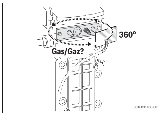
Fig. 50 Contrôle d'étanchéité
