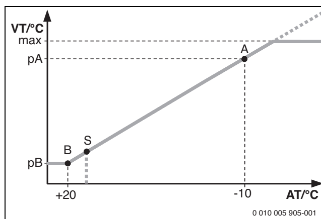
Fig. 79 Courbe de chauffe
