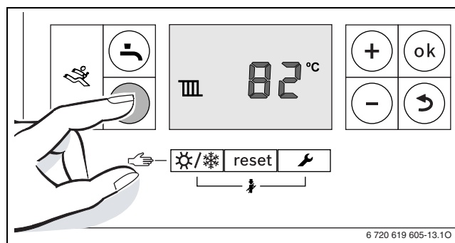
Fig. 35 Affichage température de départ
