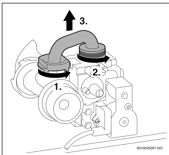
Fig. 68 Retrait du tuyau de gaz
