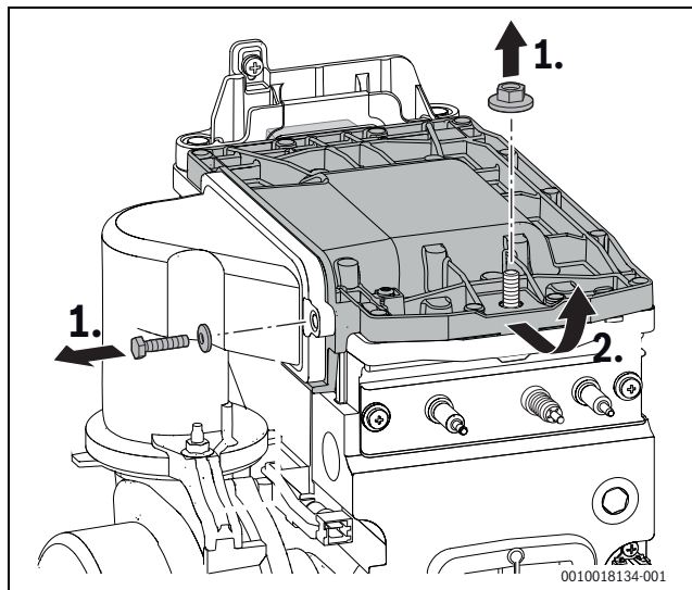
Fig. 51 Détacher le couvercle du brûleur
