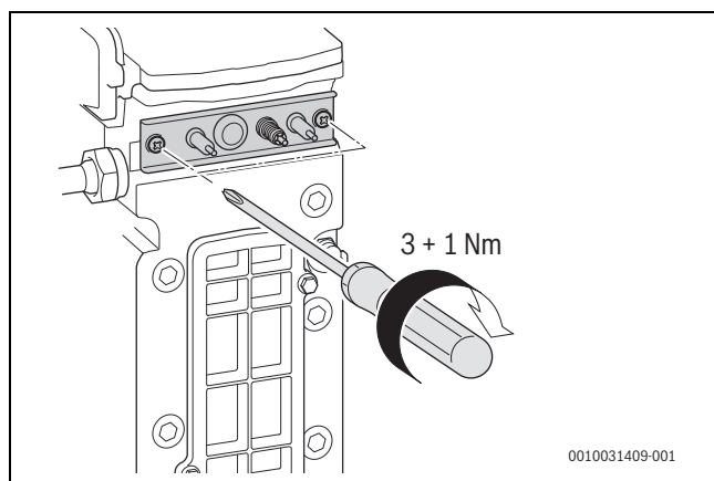
Fig. 49 Remonter le jeu d'électrodes
