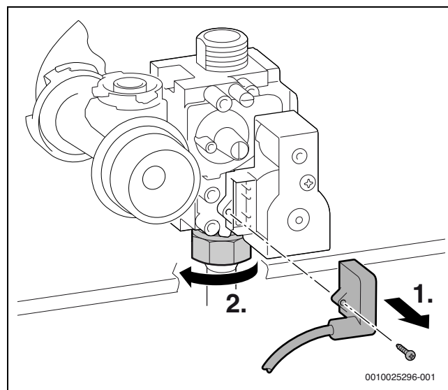
Fig. 69 Retirer le connecteur et desserrer l'écrou-raccord
